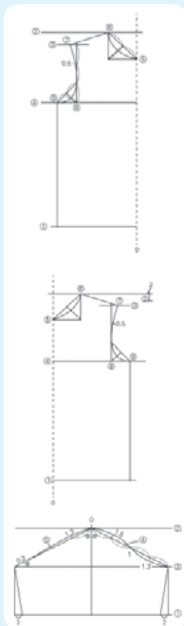
图3-36 圆领衫结构图绘制过程
