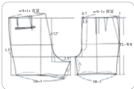
图4-7 平面裁剪
