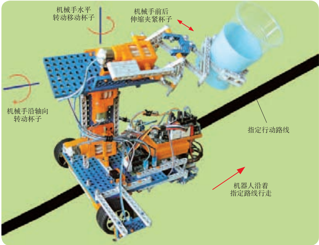
图4-22 倒水机器人的运动形式
