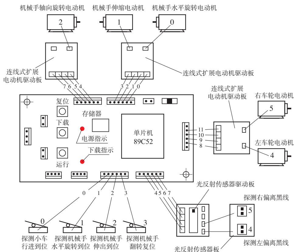
图4-28 倒水机器人控制电路连接示意图
