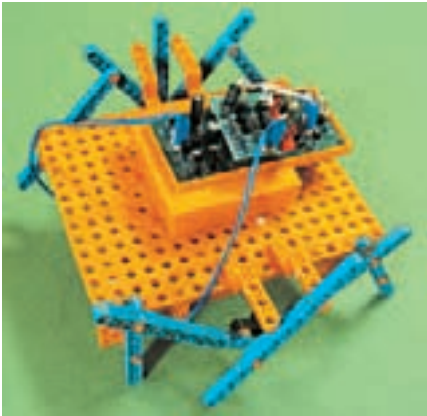
简易爬行机器人
