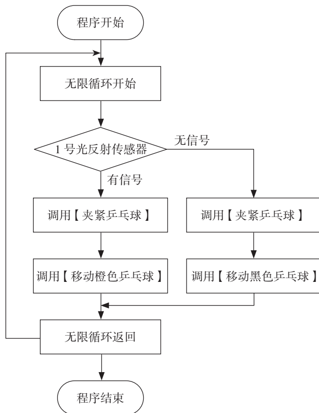
图4-12 主程序
