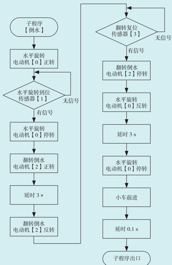
图4-35 倒水机器人“倒水”子程序
