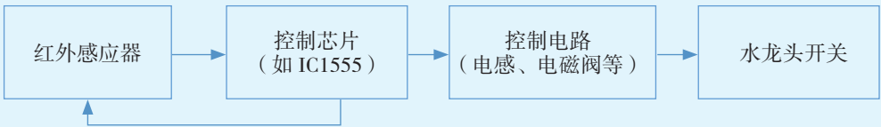
图3-6 自动感应控制水龙头控制示意图
