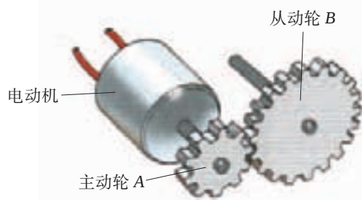
图2-3 齿轮的啮合
