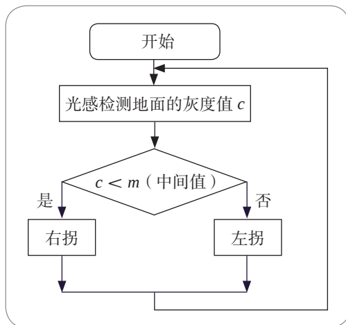
图3-29 小车的工作流程图
