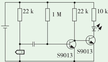
图3-3 声控灯电路图
