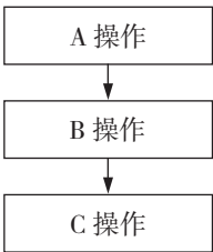
图3-23 顺序流程
