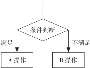
图3-24 分支结构
