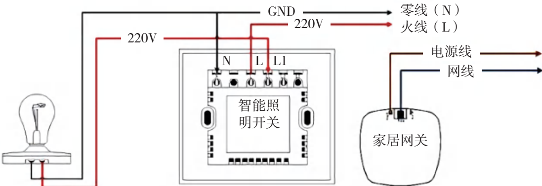
图3-33 智能照明系统连线
