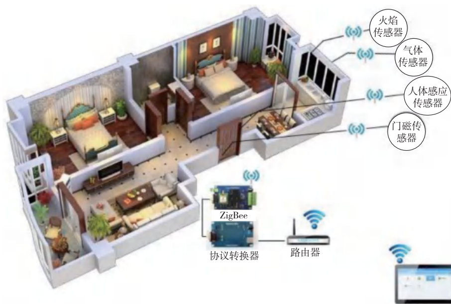
图2-11 智能安防报警系统
