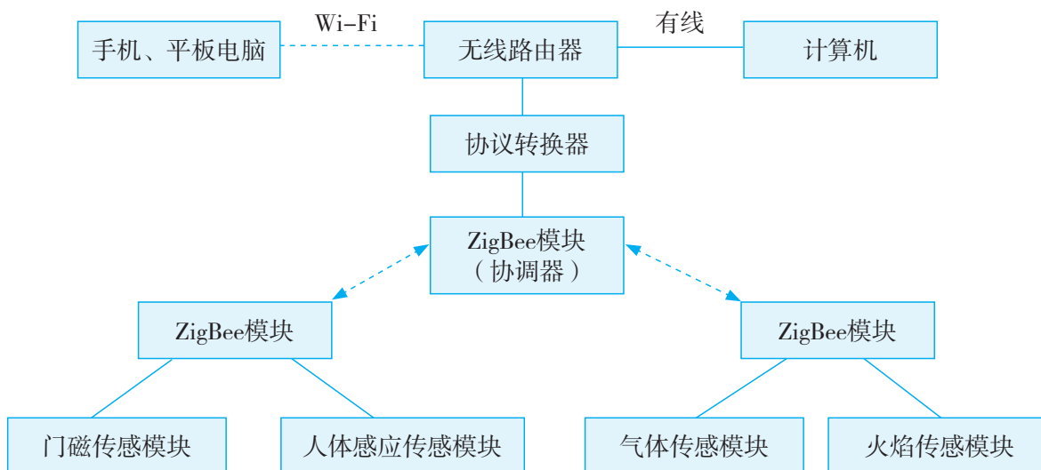
图2-12 智能安防报警系统模块通信结构
