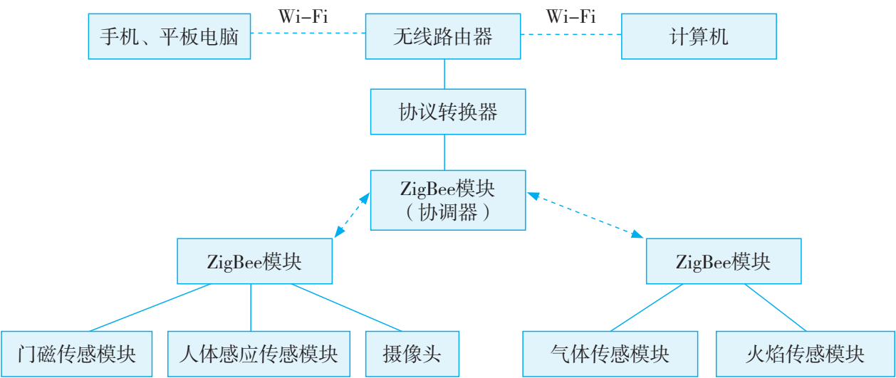
图2-13 改进后的智能安防报警系统模块通信结构
