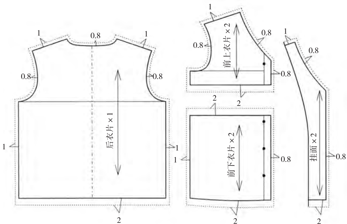
图3-20 衣片放缝
