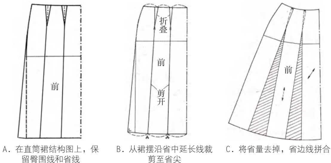
图3-13 剪切变化过程
