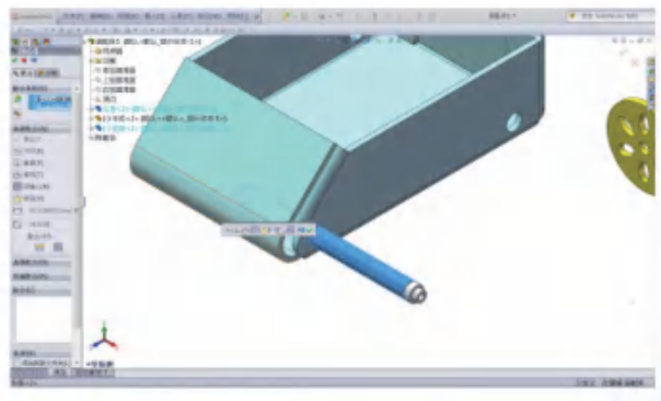
图3-36 轮轴同心定位
