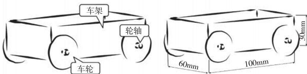
图2-11 “无碳小车”
