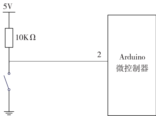
图4-13 开关与微控制器的接口电路
