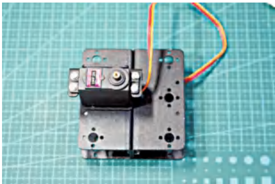
图2-48 安装舵机
