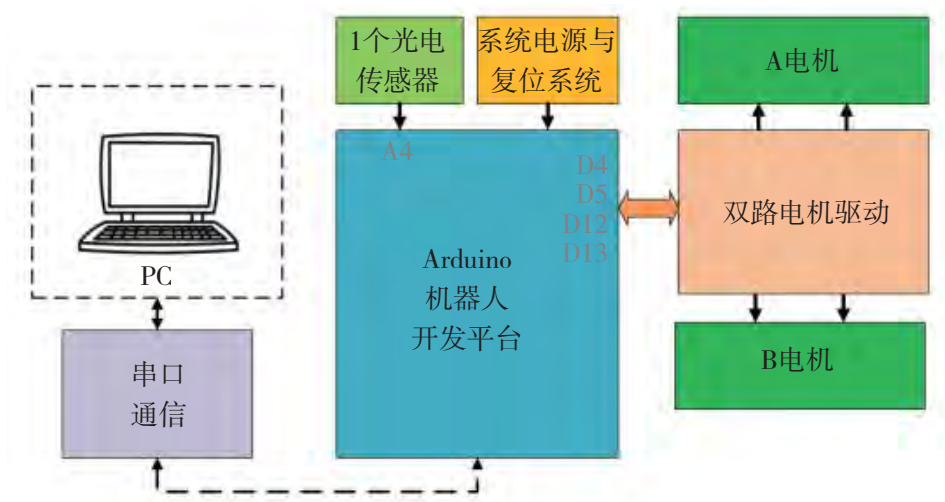
图5-27 系统框架与主要引脚连接
