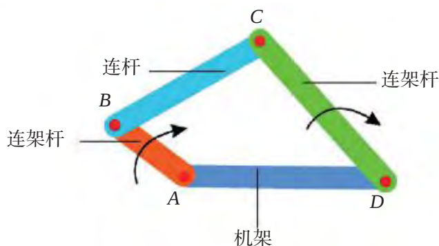
图2-18 铰链四连杆机构
