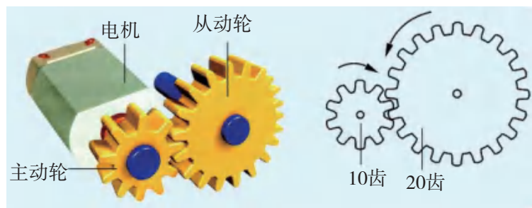
图2-8 电机驱动的直齿圆柱齿轮传动装置
