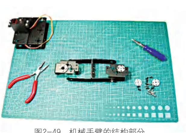
图2-49 机械手臂的结构部分
