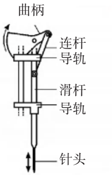
图2-23 缝纫机的针头机构
