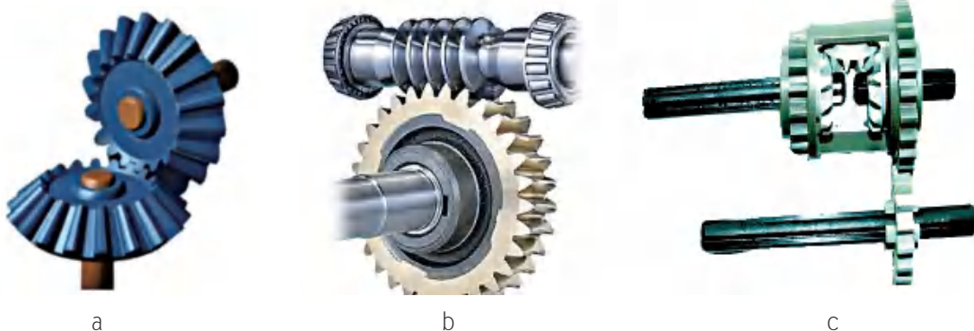
图2-13 机器人中的传动装置
