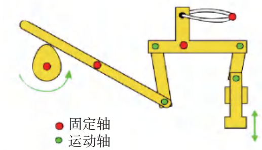
图2-25 凸轮和平面连杆组成的机构
