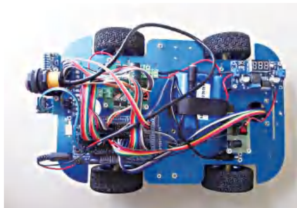
图2-2 机器人小车
