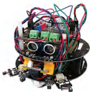
图2-28 固定形式的机器人
