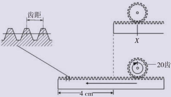
图2-12 齿条与齿轮运动转换示意
