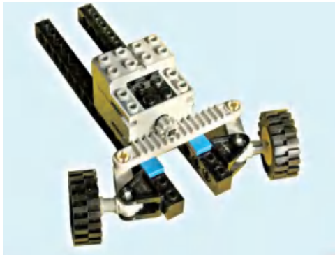
图2-11 机器人中的齿条与齿轮
