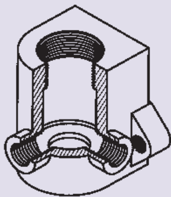
图2-52 泵体立体图
