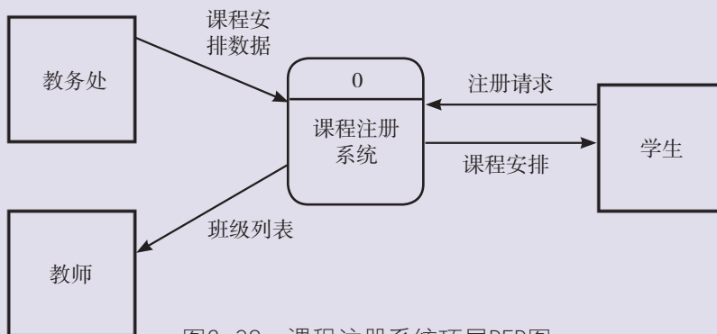
图2-38 课程注册系统顶层DFD图
