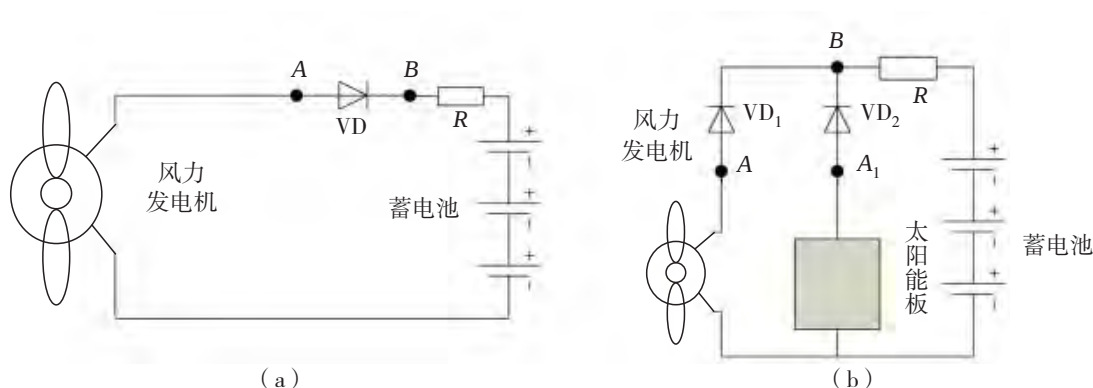
图4-25 风光互补供电装置的简易充电电路
