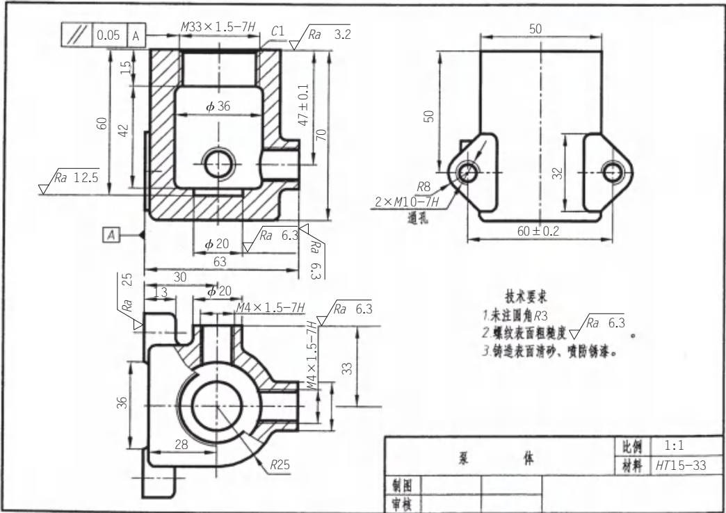
图2-49 泵体零件图
