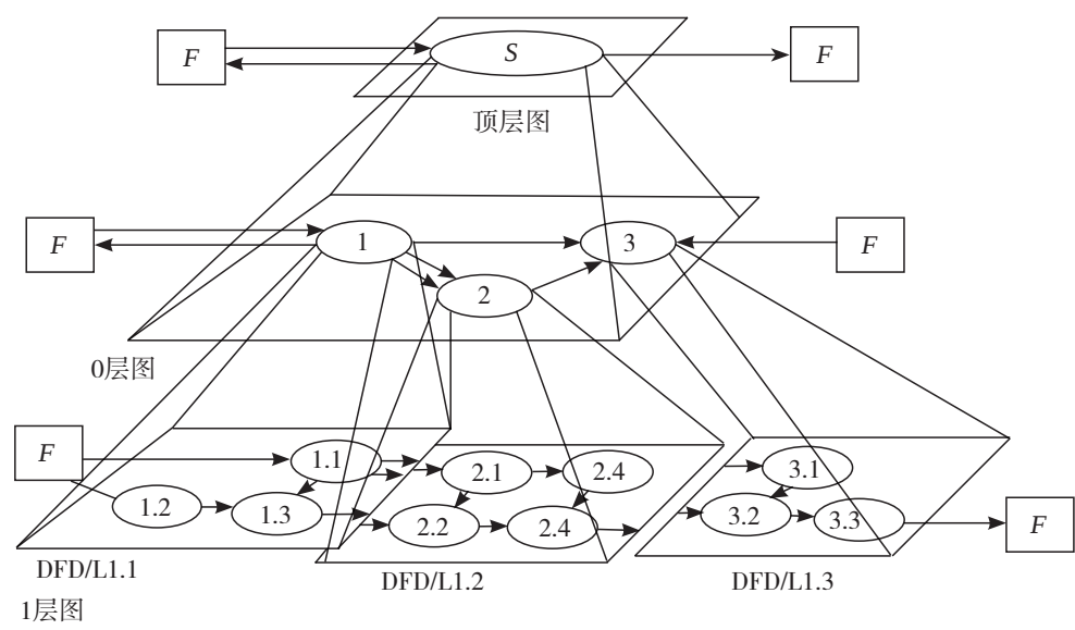
图2-37 数据流图的层次
