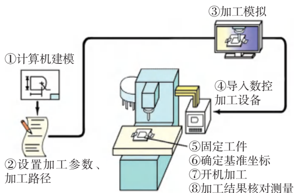
图4-6 数控加工的主要过程示意
