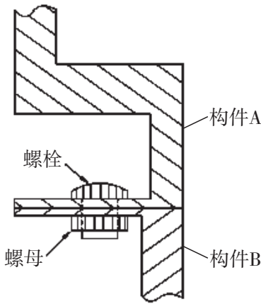
图2-4 金属部件示意图
