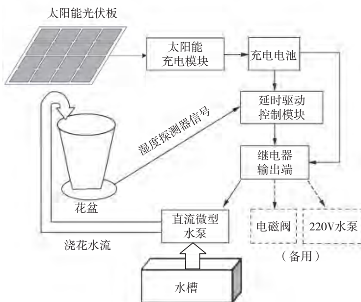
图2-6 太阳能自动浇花系统
