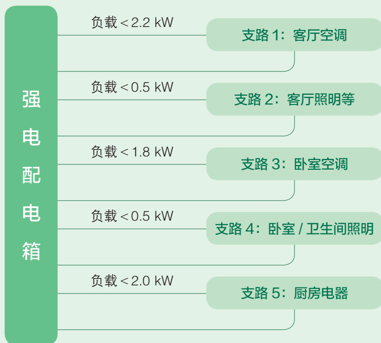
图3-15 强电系统各支路方案
