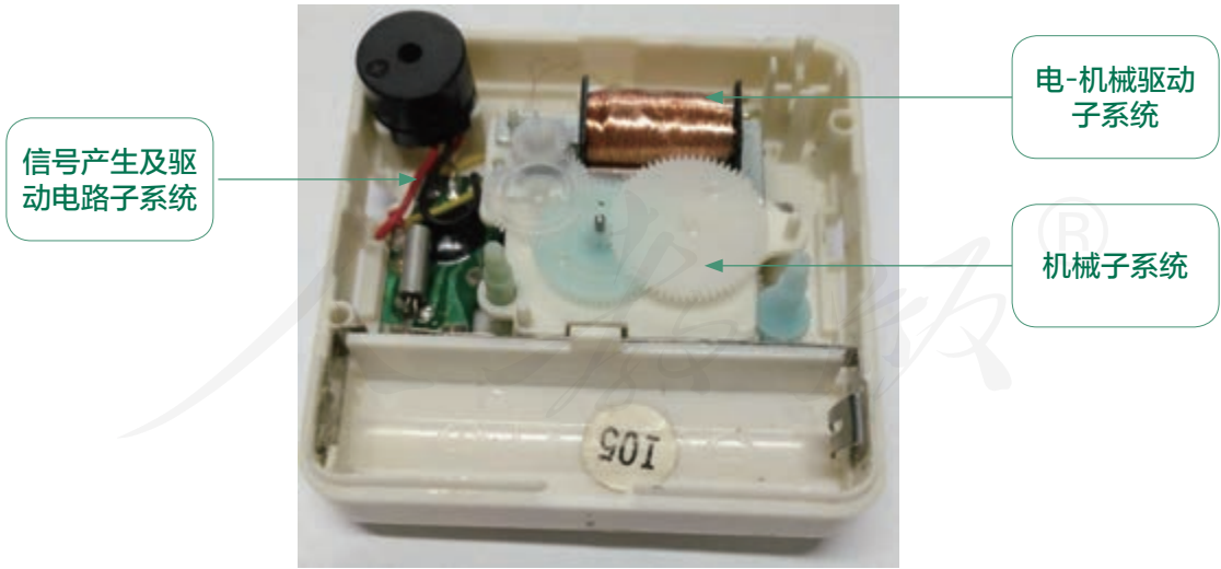
图3-8 指针式石英表的实物图
