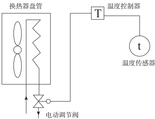
图4-19 空调温度控制系统示意图
