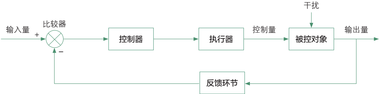
图4-18 闭环控制系统的干扰情况
