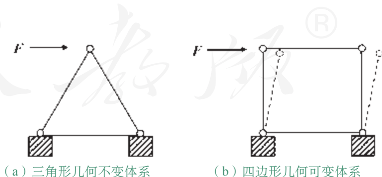
图 1-25 结构的形状与稳定性
