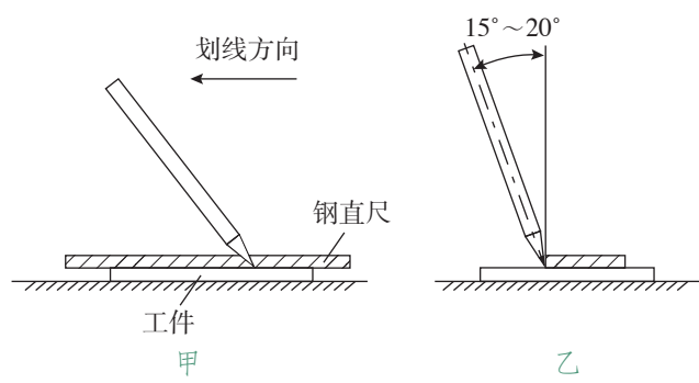
图3-16 针尖位置
