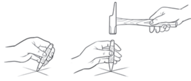
图3-17 样冲的用法
