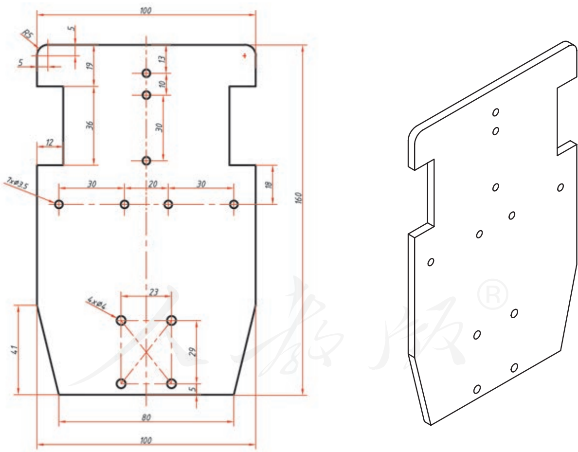
图2-69 循迹小车底板
