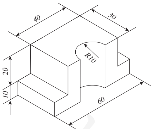
图2-54 物件形体图1
