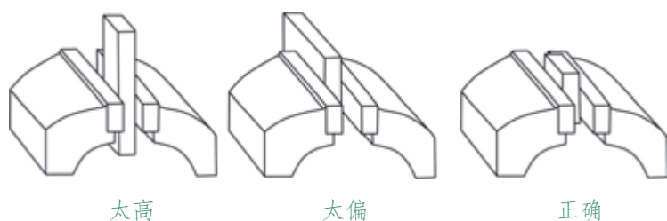
图3-30 工件装夹
