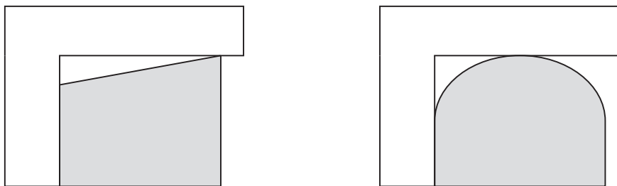
图3-35 不合格锉面
