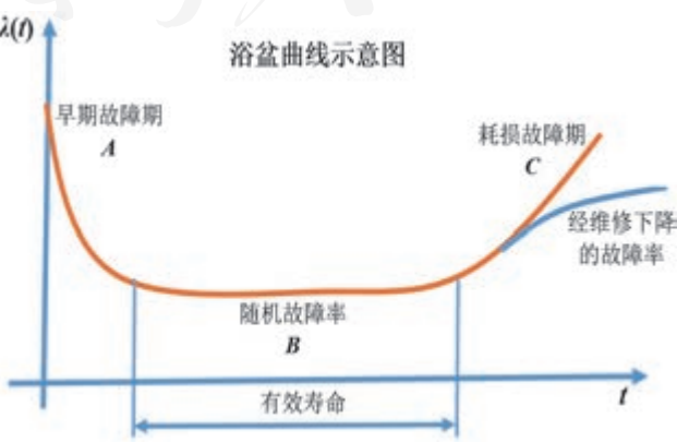
图4-19 典型故障曲线（浴盆曲线）示意图
