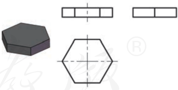
图2-52 平放六棱柱三视图
