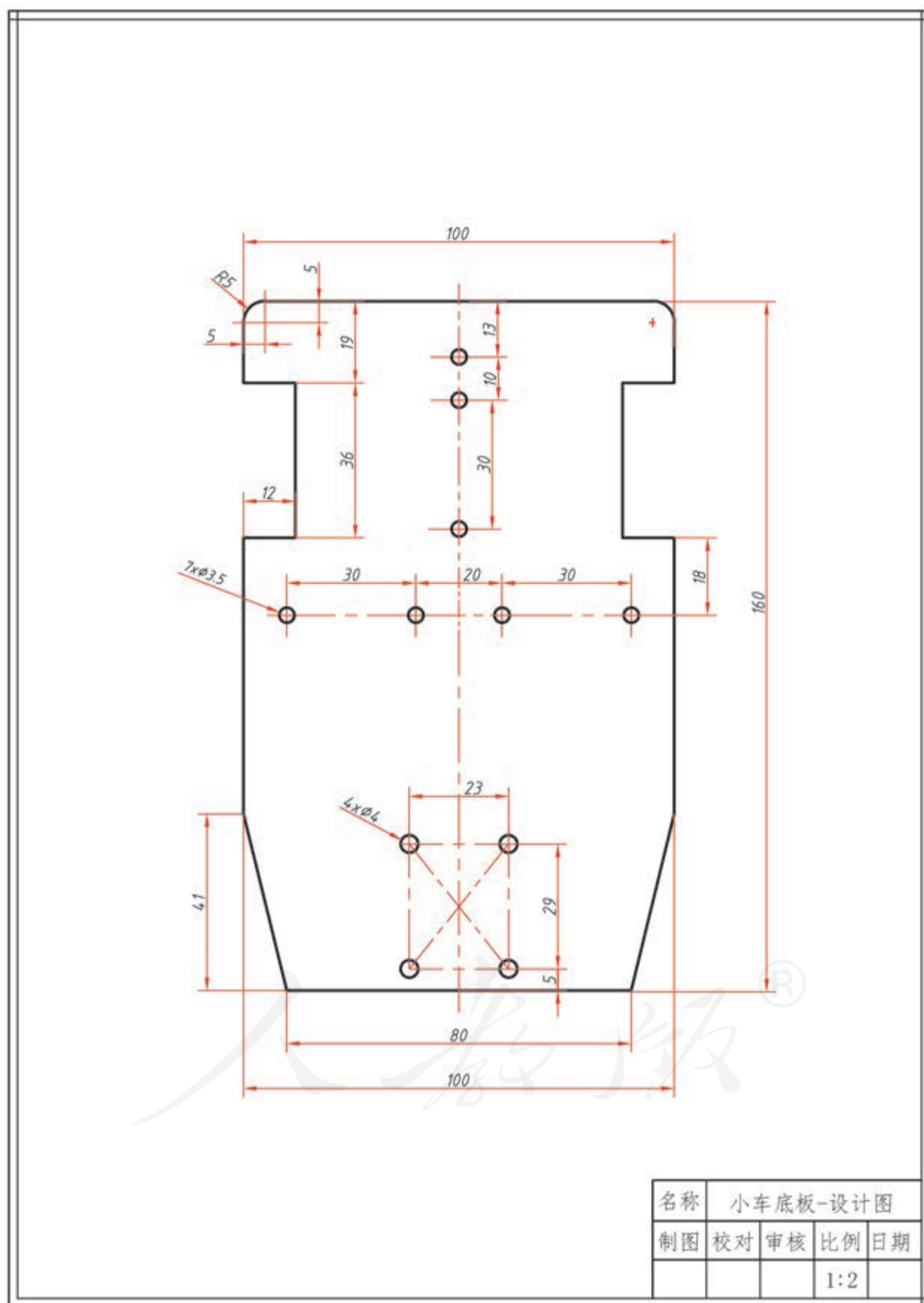
图2-77 循迹小车底板设计图
