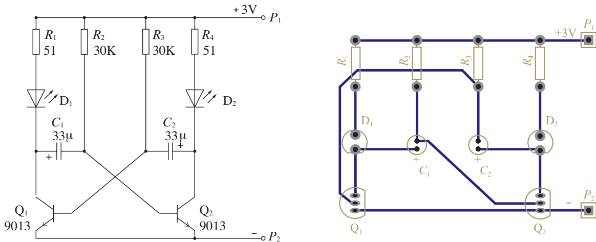
图3-51 简易双闪光灯电路
