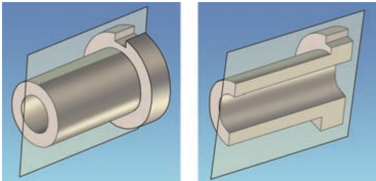
图2-60 剖视图形成过程
