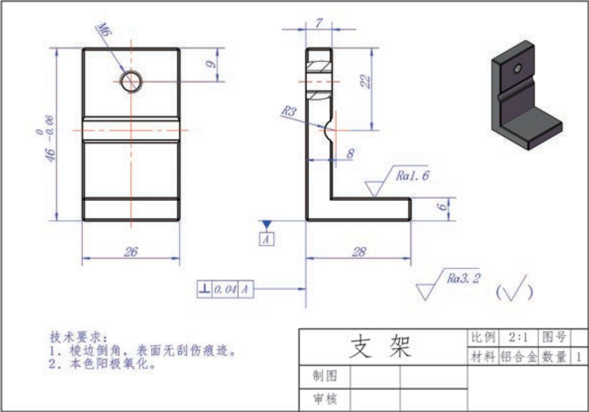
图2-34 支架零件图
