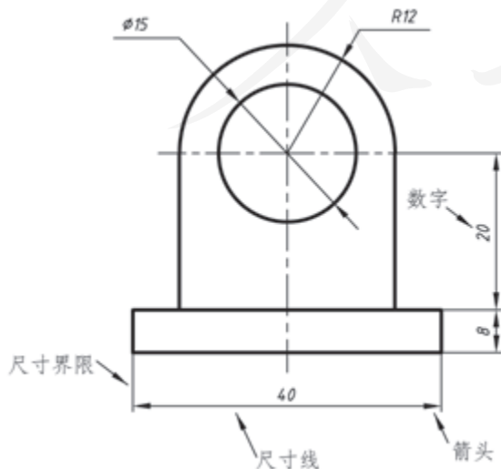
图2-63 尺寸标注
