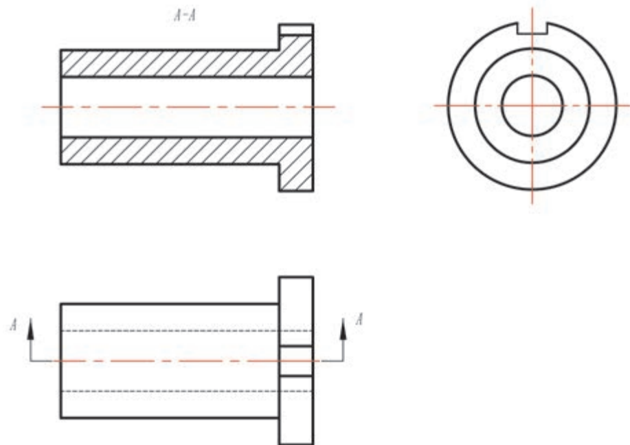
图2-62 零件剖视图
