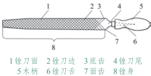
图3-29 锉刀的构造
