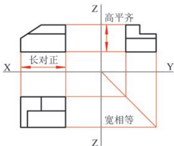
图 2-49 三视图投影规律
