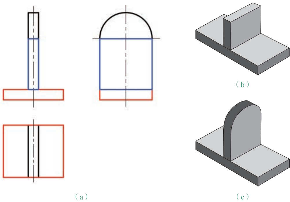
图2-58 识读三视图
