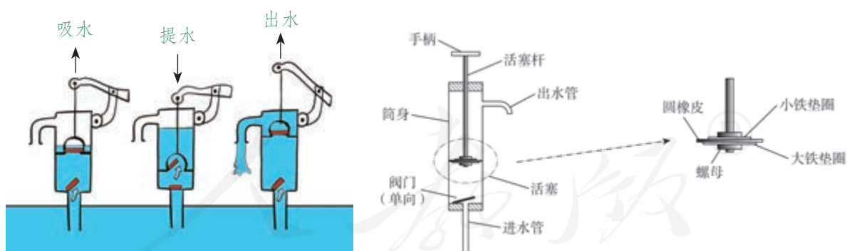
图 1-17 活塞式抽水机
