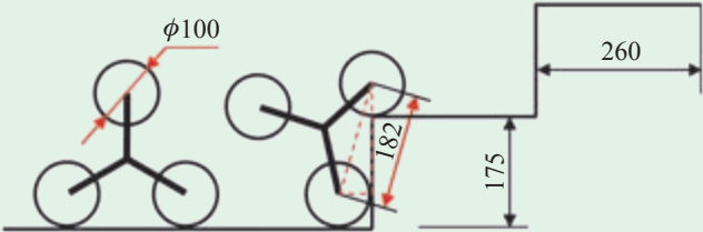
图 2-5 车轮功能图
