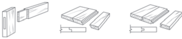
图3-13 拼接和插接
