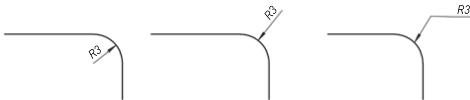
图2-65 半径标注
