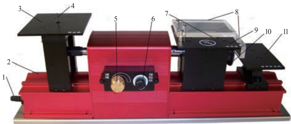
1 直流电源线 2 导轨 3 锯平台 4 锯条 5 调速开关 6 保险丝 7 砂圈 8 防护罩 9 平面磨平台 10 砂皮 11 侧面磨平台
