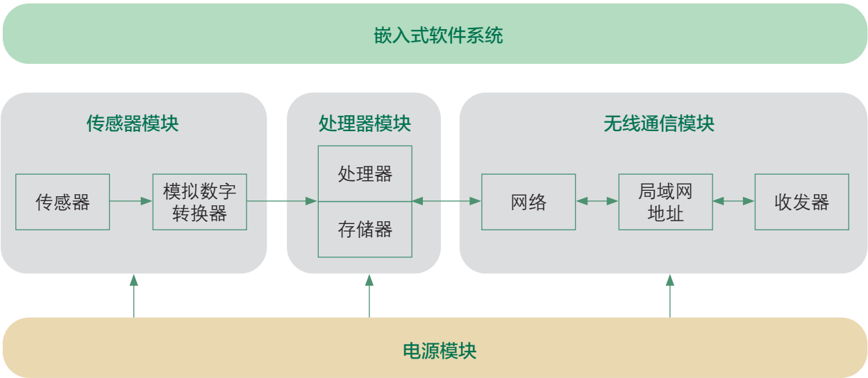
图2-3 无线传感网络节点的体系结构
