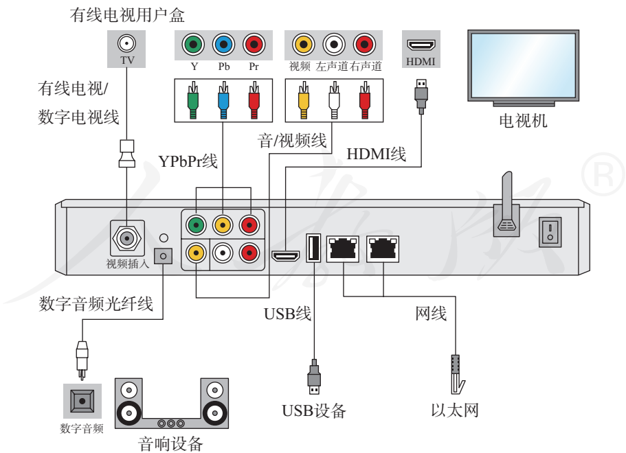
图1-16 家用电器接口
