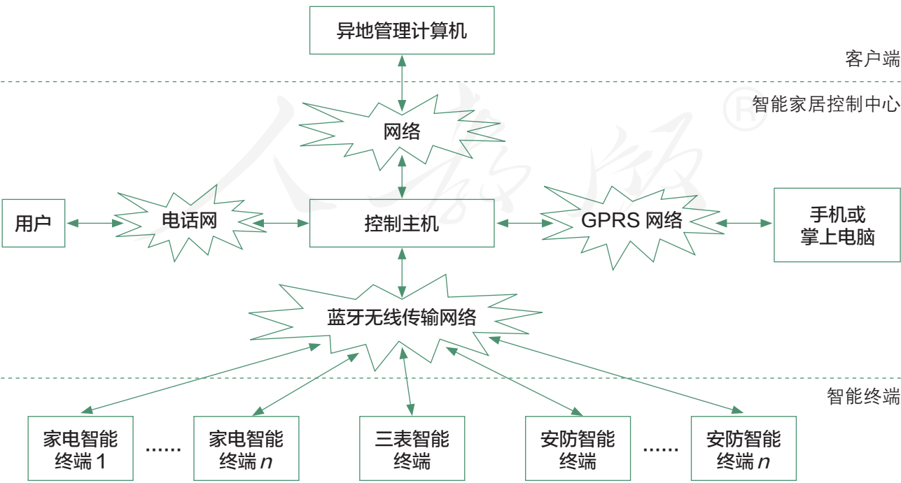
图4-1 智能家居系统的总体架构与终端控制主机
