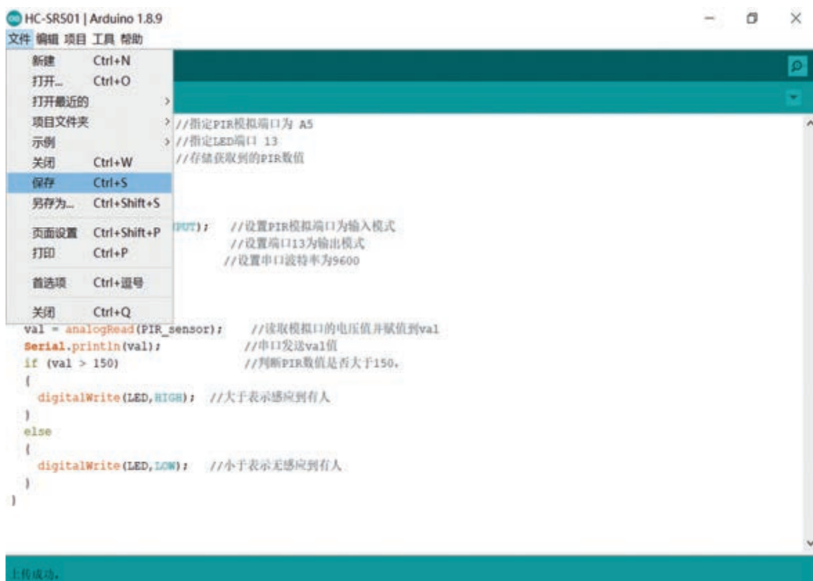
图 3-23 人体感应灯编译保存的软件界面
