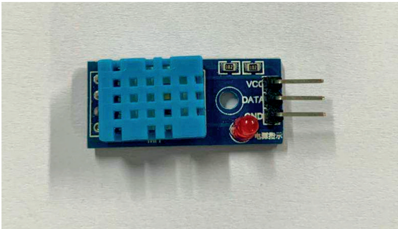
图3-14 DHT11实物
