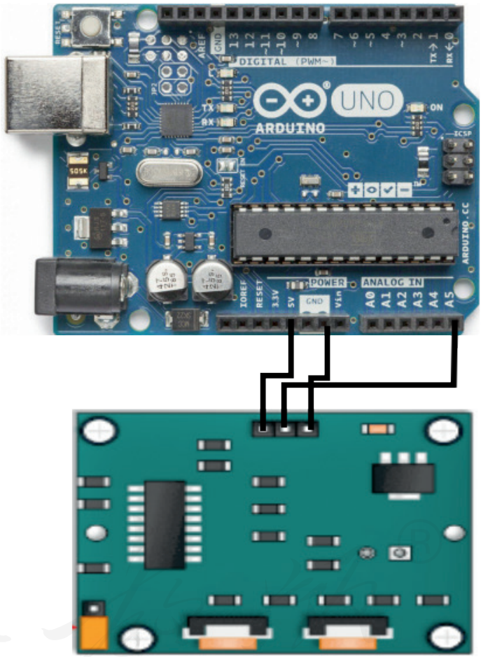
图3-22 系统接法
