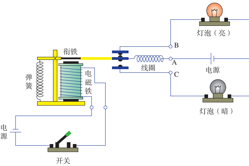
图3-1 继电器原理
