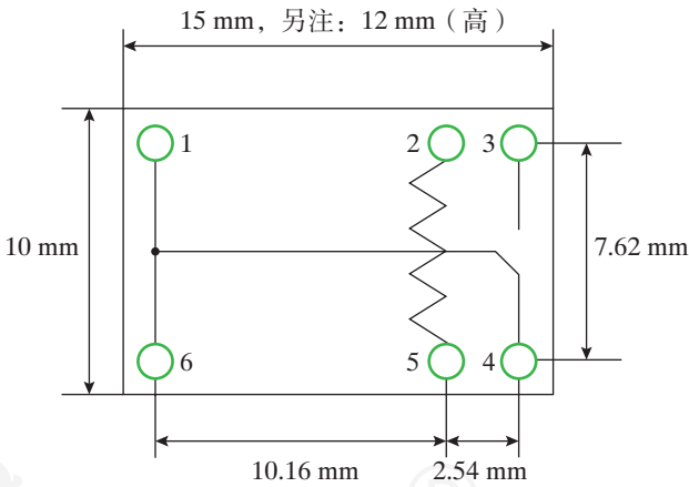
图3-3 继电器封装引脚（底视图）
