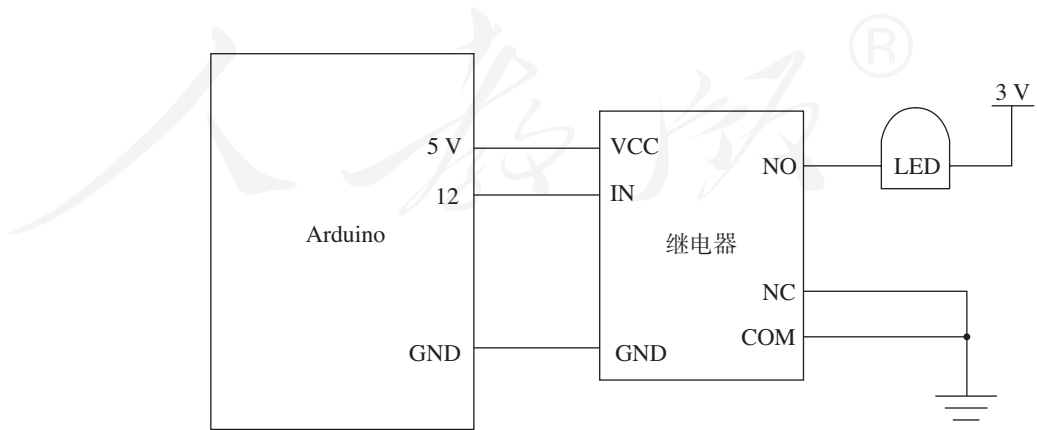
图3-4 继电器与单片机相连控制电路
