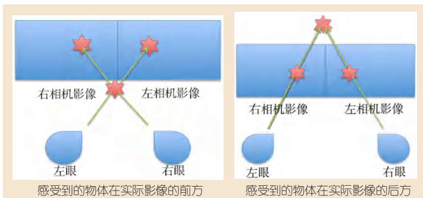
双眼视差产生立体空间感图示
