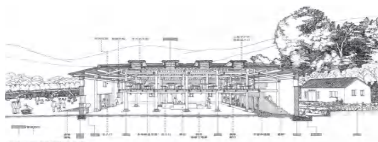
▲ 徽派古村——奇峰村史馆（2018年）素朴建筑工作室/清华大学建筑学院
