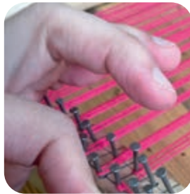
② 以S形状将毛线缠绕在综框两边的齿梳木条上。其中经线要绷紧，为下一步做好准备。
