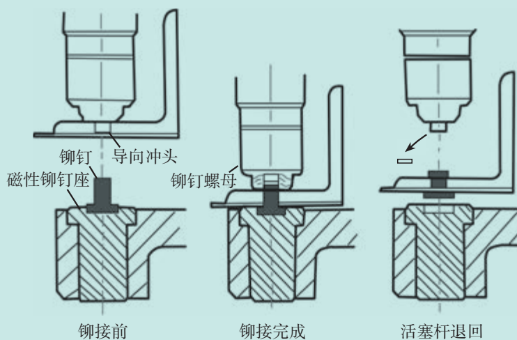
◇ 铆接步骤示意图
