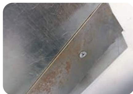
5. 将钉子插入两片金属板的钻孔中，压紧 6. 铆接完成。
