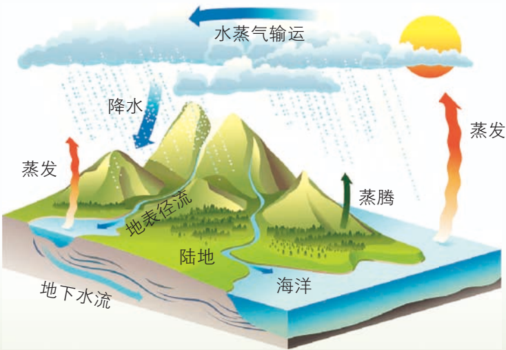
图 3-14 水循环示意图
