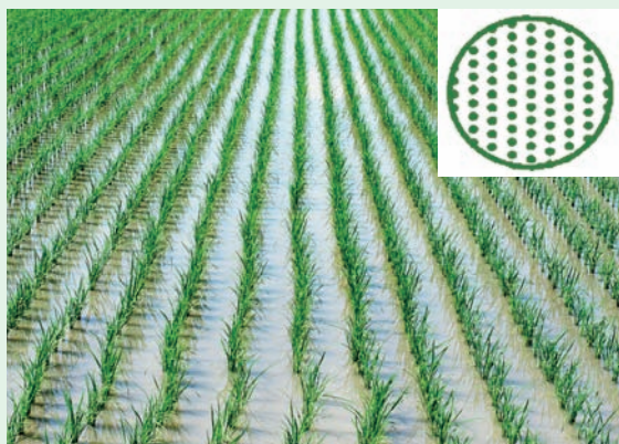
B. 均匀分布
