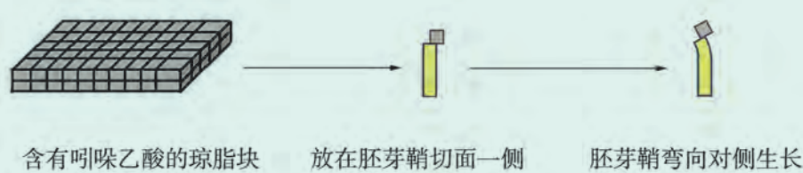
图 5-8 郭葛实验示意图
