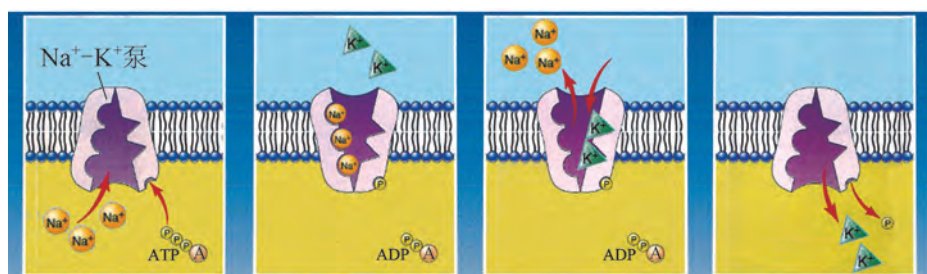
图 2-14 \text{Na}^+-\text{K}^+ 泵示意图
