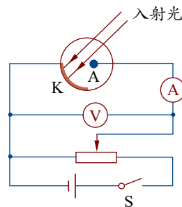
图 6-3 研究光电效应的电路图
