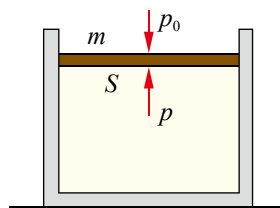
图 1-19 分析气缸内气体压强的示意图
