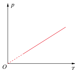
图 1-27 p-T 图像
