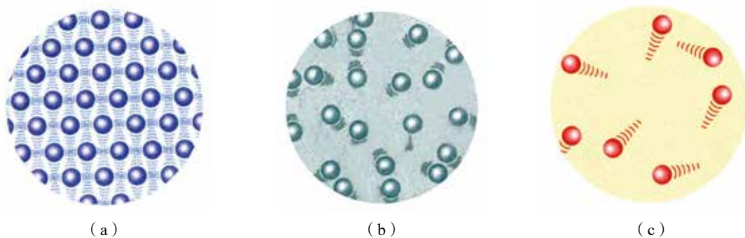
图 1-8 固体、液体、气体分子的运动示意图
