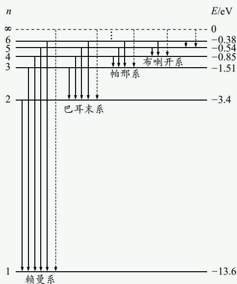
图 4-18 氢原子谱线系示意图
