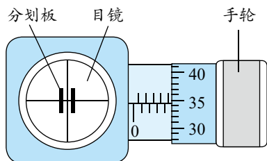
图 5-12 测量头示意图
