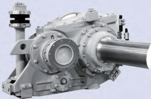
图 2-1-8 高铁列车齿轮传动系统（部分）
