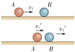
图 1-4-2 两球的碰撞
