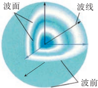
图 3-4-1 球面波
