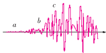
图 3-3-2 地震波示意图
