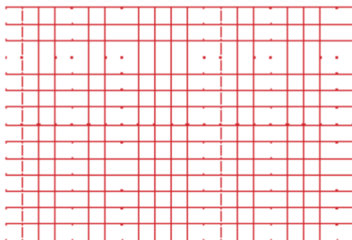
图 2-4-3 坐标纸
