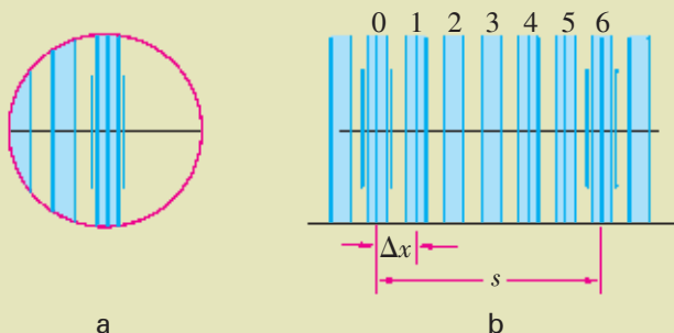
图 4-4-1 测量条纹的间距
