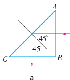
图 4-2-4 全反射棱镜
