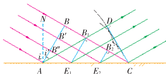
图 3-4-6 波的反射
