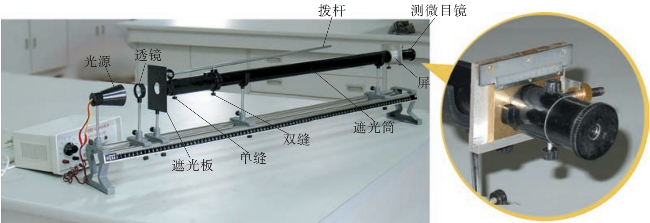
图 4-3-1 双缝干涉仪
