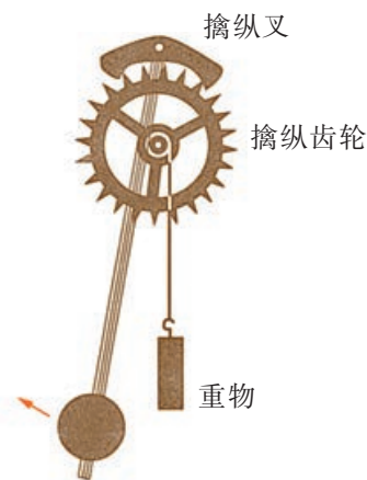
图 2-5-4 摆钟的擒纵齿轮和擒纵叉
