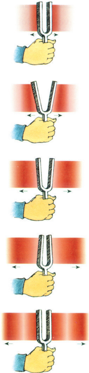
图 3-1-6 声波是纵波
