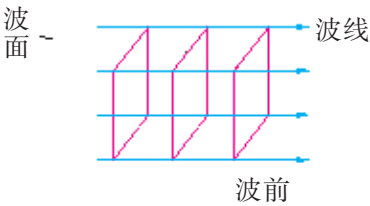
图 3-4-2 平面波
