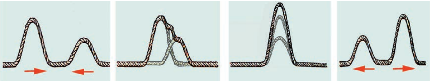
图 3-5-2 绳波的叠加
