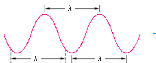
图 3-2-2 波长
