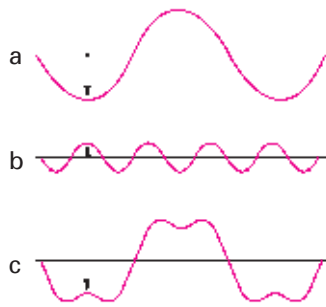
图 2-1-10 振动合成示意图
