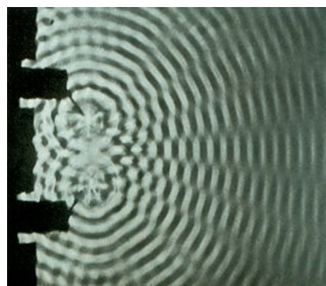
图 3-5-5 水波干涉图样
