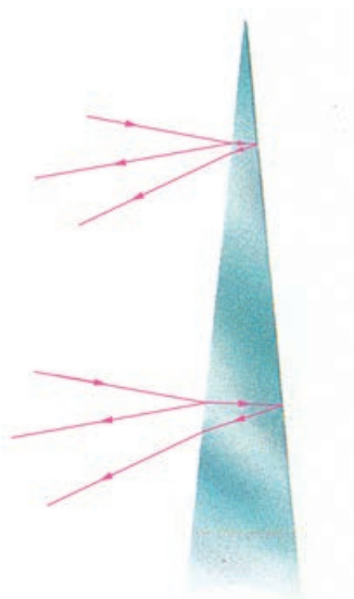
图 4-3-8 液膜前后两个面反射光的干涉
