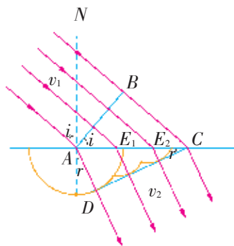
图 3-4-9 波的折射
