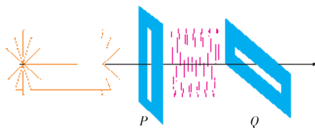
图 4-6-6 偏振光不能通过偏振片 Q
