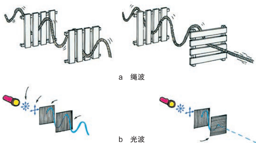
图 4-6-4 横波通过狭缝的情况
