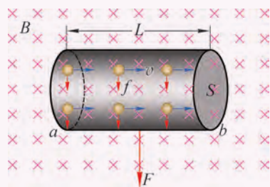
图 5-22 导线内运动电荷的洛伦兹力宏观表现为安培力
