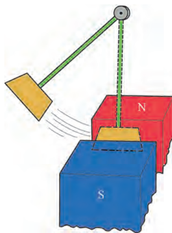
图 7-6 电磁阻尼现象
