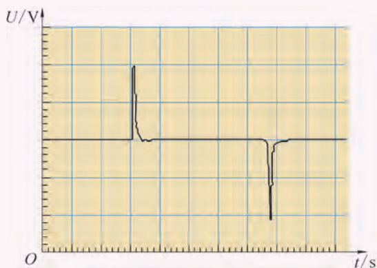
图 9-19 电压-时间图像
