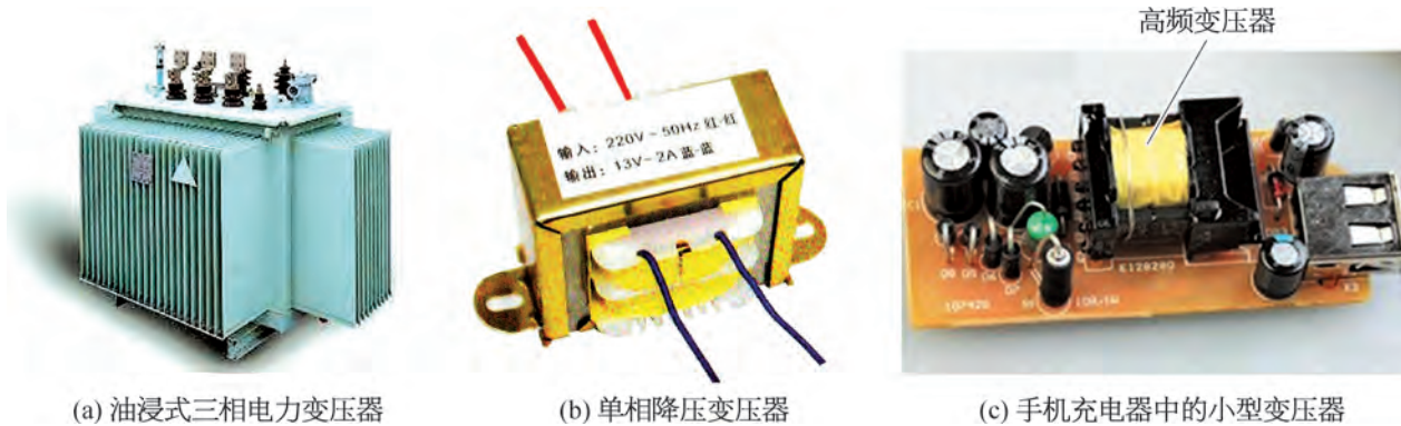
图 7-24 常见的变压器
