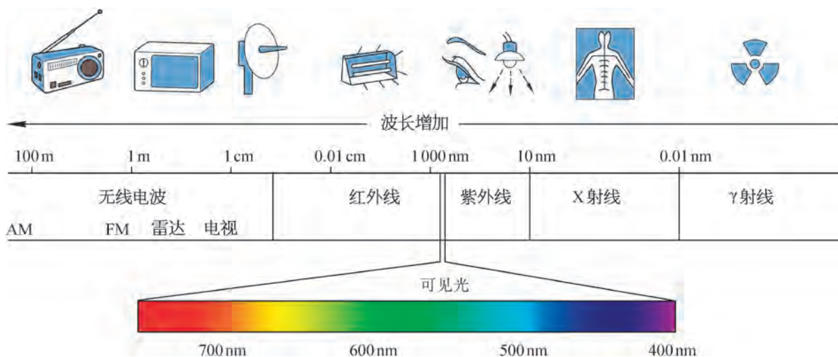
图 8-21 电磁波谱
