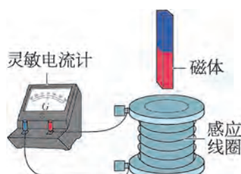
图 6-3 研究感应电流的方向的实验装置
