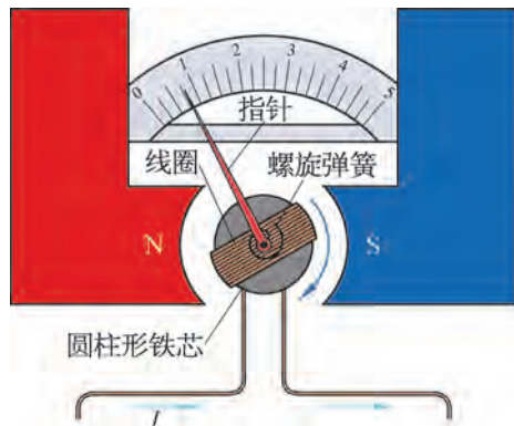
图 5-10 磁电式电表的基本结构图
