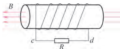
图 6-18 螺线管内产生感应电流
