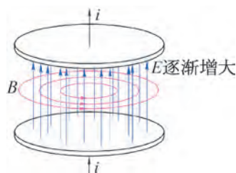
图 8-3 变化的电场产生磁场
