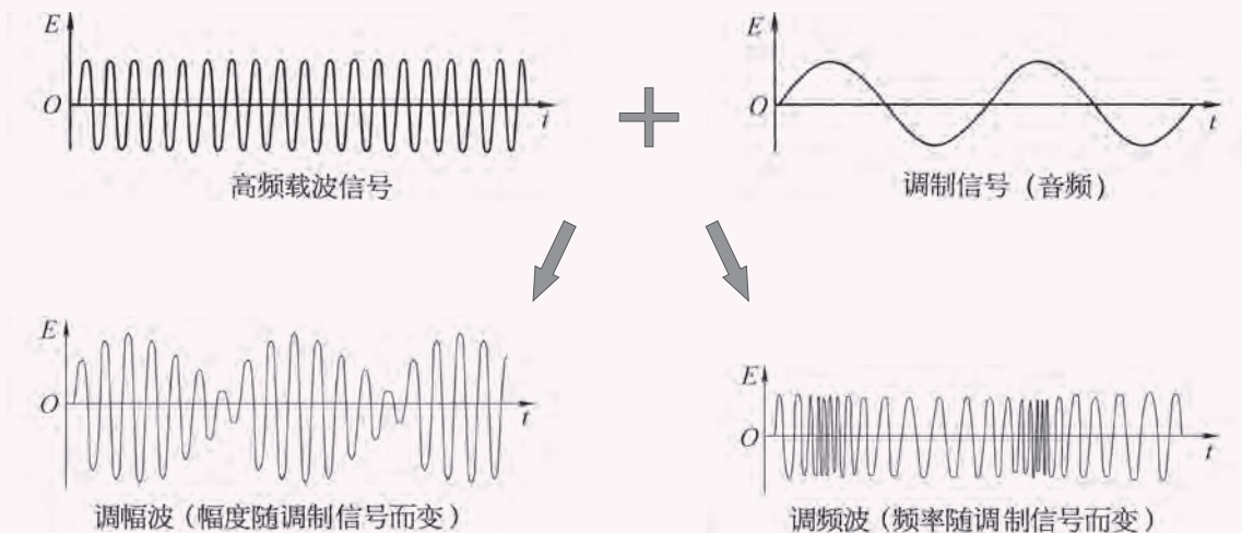
图 8-18 模拟调制示意图
