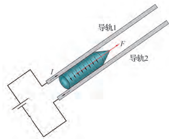
图 5-13 电磁炮原理图
