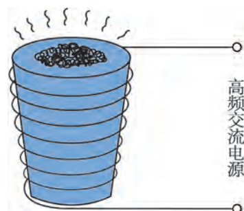
图 7-5 高频感应炉示意图
