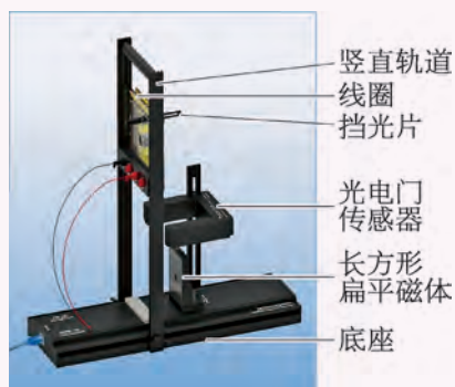
图 6-20 研究感应电动势与线圈运动速度间的关系
