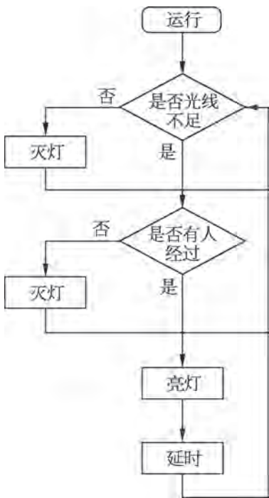
图 9-25 自动控制路灯装置程序逻辑图
