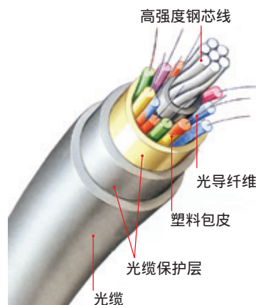
▲ 图4-3-8 光缆的结构
