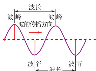
▲ 图3-2-1 横波的波长
