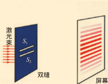
▲ 图4-4-2 双缝干涉实验
