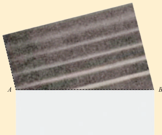
▲ 图3-4-6 机械波射到两种介质界面
