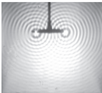
▲ 图3-5-3 水波的干涉
