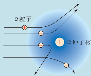
▲ 图1-5-12 金原子核对α粒子的散射
