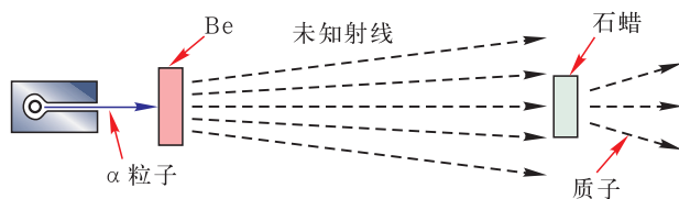
▲ 图1-5-5 α粒子轰击轻金属铍
