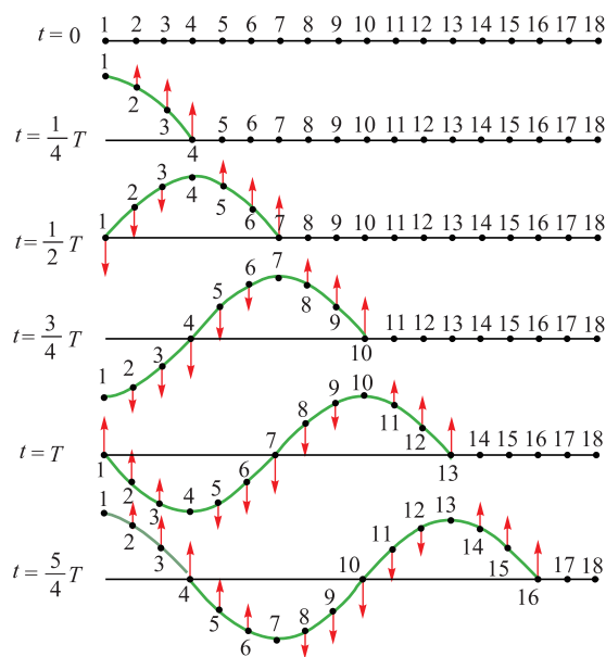
▲ 图3-1-4 绳波的形成
