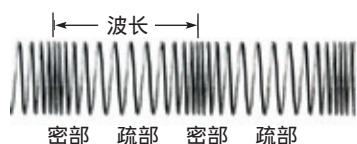
▲ 图3-2-2 纵波的波长
