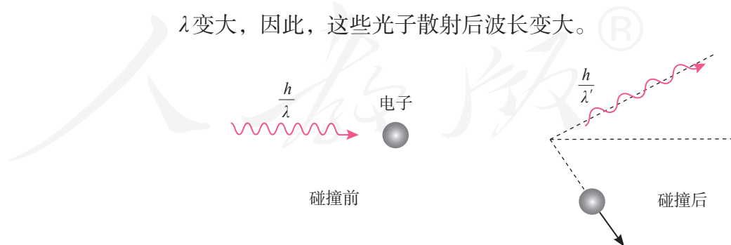
图 4.2-6 光子既有能量也有动量
