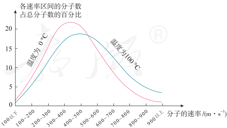
图1.3-2 氧气分子的速率分布图像
