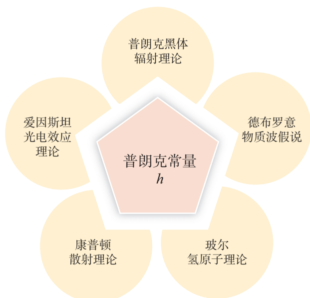
图 4.5-3 一系列理论都和普朗克常量紧密相关 们需要建立描述微观世界的物理理论。
