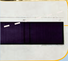
乙 夫琅禾费记录太阳光谱
