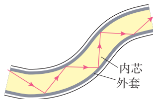
图 4.2-7 光导纤维
