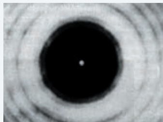
图 4.5-6 泊松亮斑
