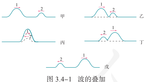
图 3.4-1 波的叠加
