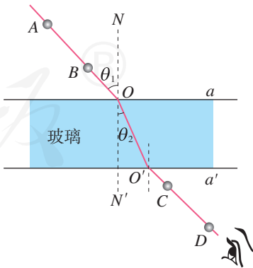
图 4.1-3 测量玻璃的折射率
