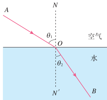
图 4.1-2 光的折射
