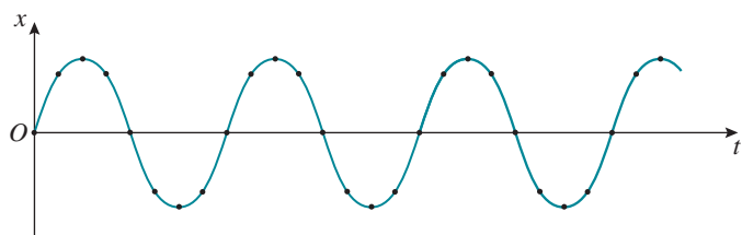
图 2.1-3 振动图像
