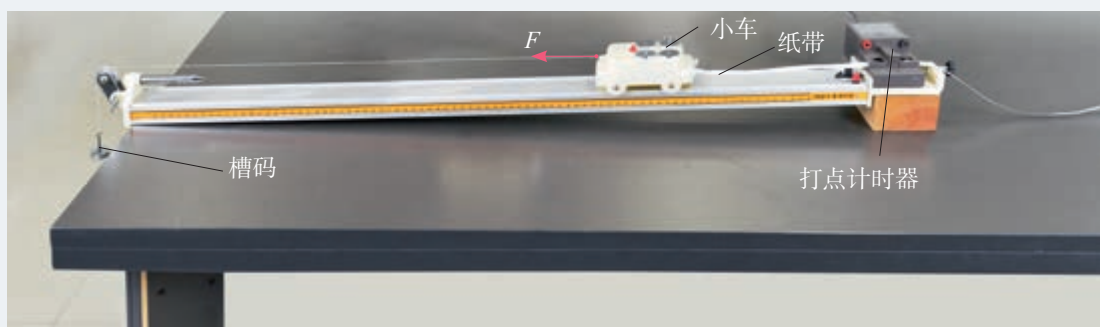
图4.2-2 实验装置
