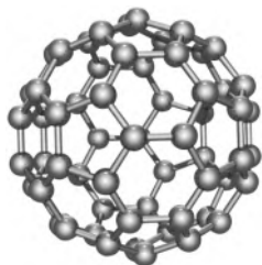
C_{60} 模型
