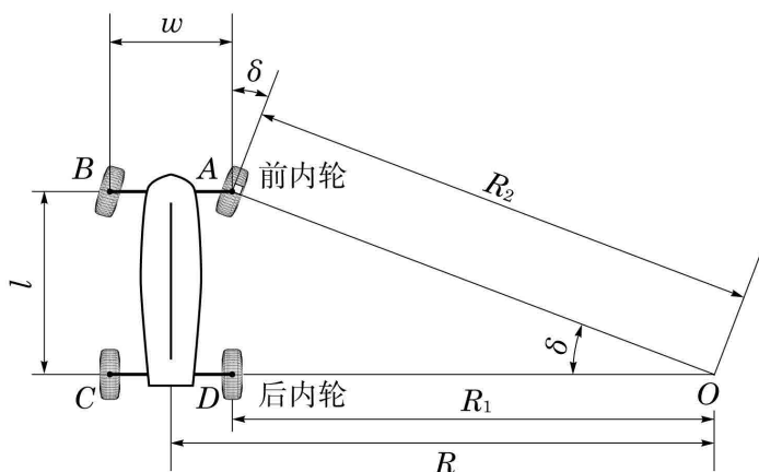
图 3-3 车辆内部图
