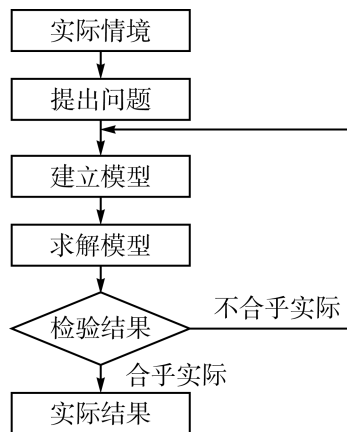
图 0-1 数学建模活动过程图示
