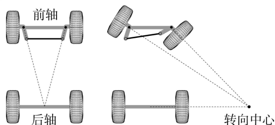
图 3-1 阿克曼转向几何原理
