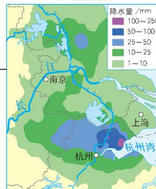
2018年8月3日上海及周边地区降水量分布 1:8 000 000
