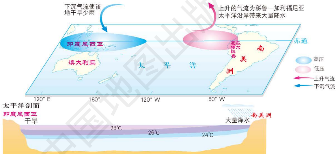
厄尔尼诺年赤道附近太平洋地区的海气状况
