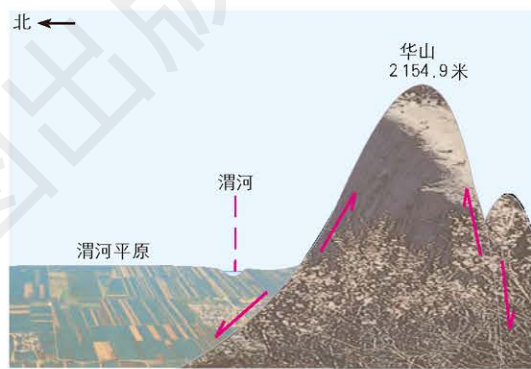
华山（断块山）、渭河平原形成示意
