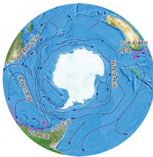
南极附近绕极环流
