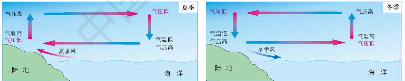
海陆热力差异导致的季风环流及其成因示意
