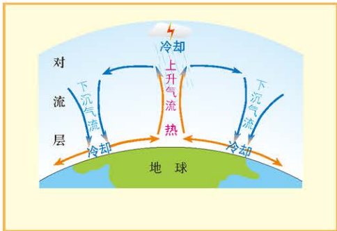
对流层大气的特点
