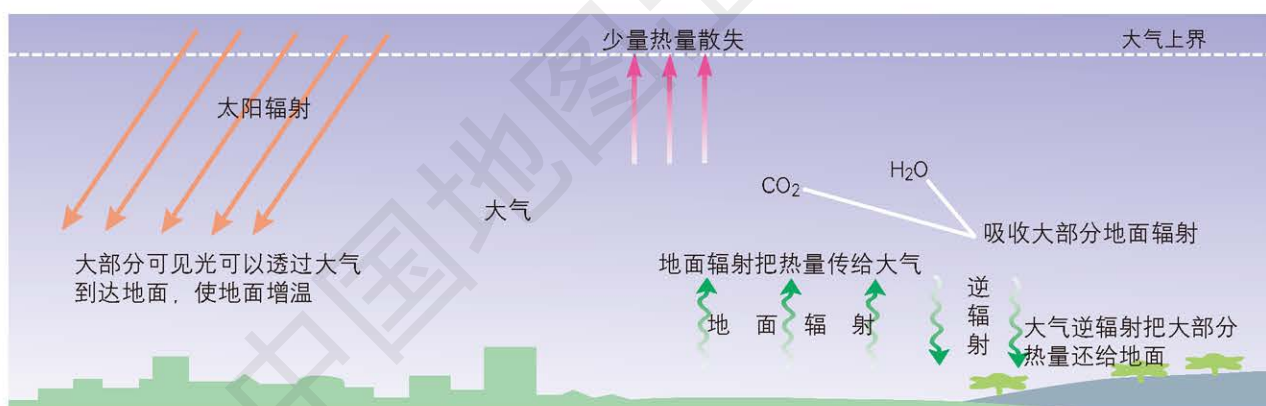
大气对地面的保温作用
