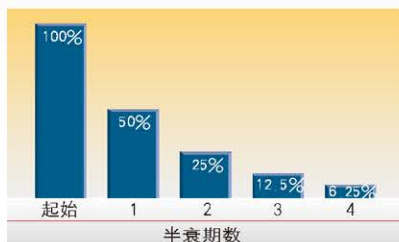
放射性元素的衰变
