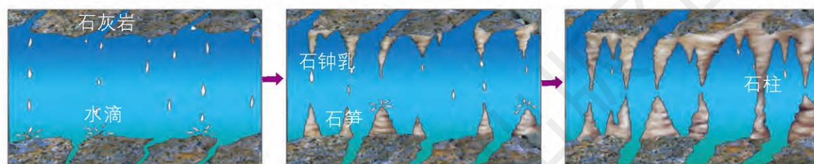
石钟乳、石笋和石柱的形成过程
