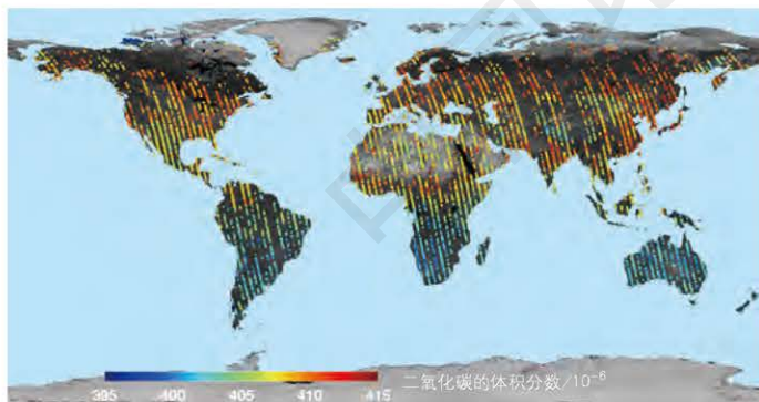
全球二氧化碳含量分布（2017年4月）
