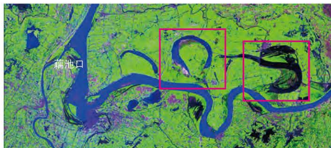
2001年长江藕池口以下河段遥感影像
