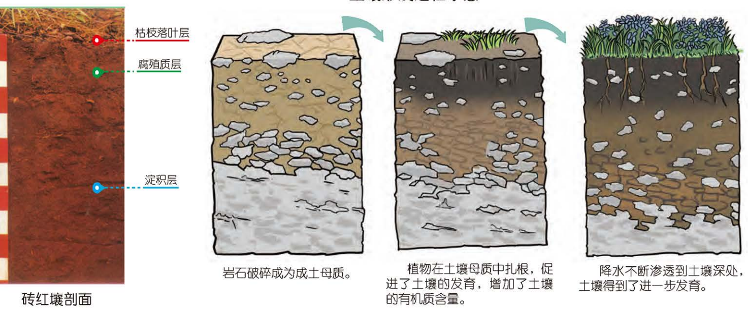
土壤形成过程示意
