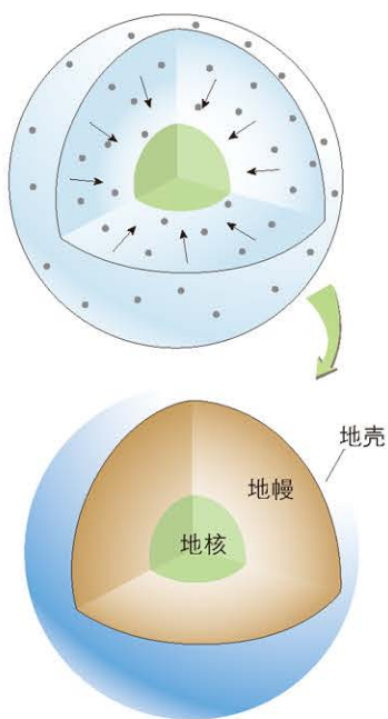
地球内部圈层形成示意
