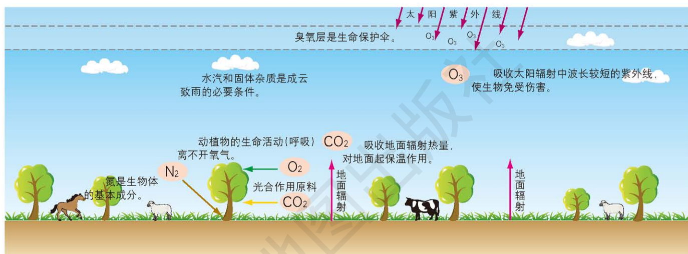
大气主要成分的作用
