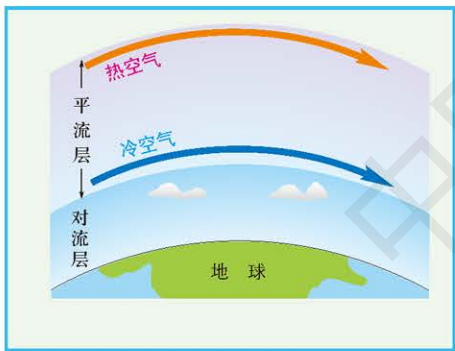
平流层大气的特点
