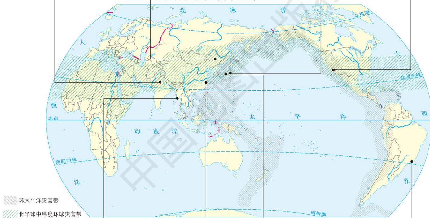
世界自然灾害带分布 1:200 000 000
