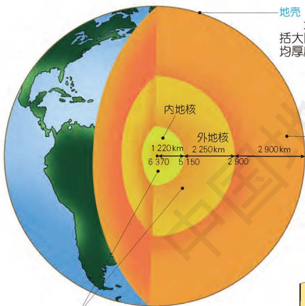
地球的内部圈层结构
