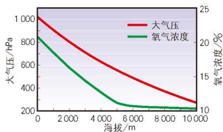
气压和氧气浓度随海拔高度的变化
