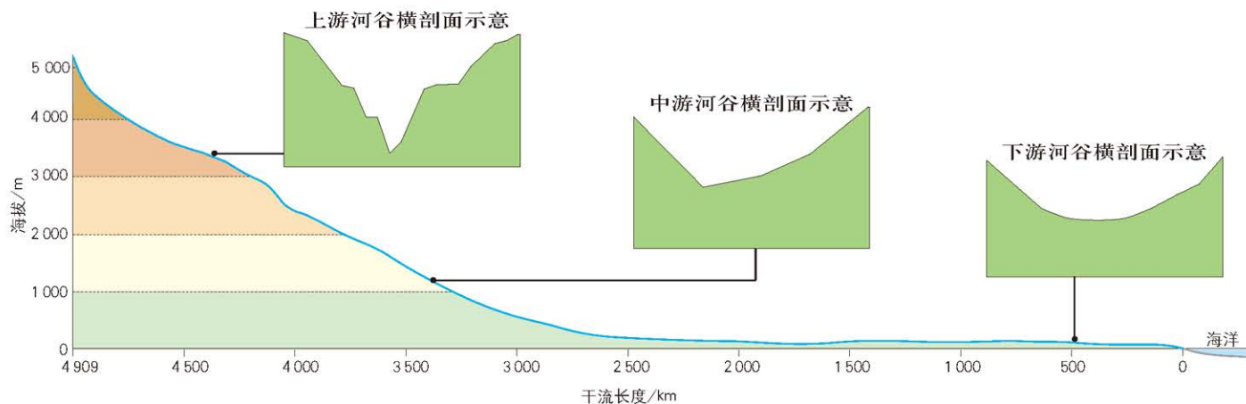
澜沧江—湄公河剖面示意
