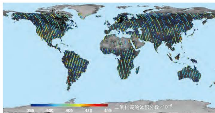
全球二氧化碳含量分布（2017年7月）
