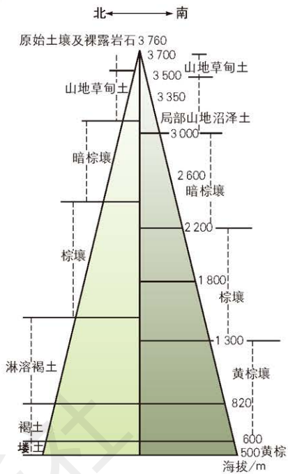
秦岭南北坡土壤垂直带谱比较
