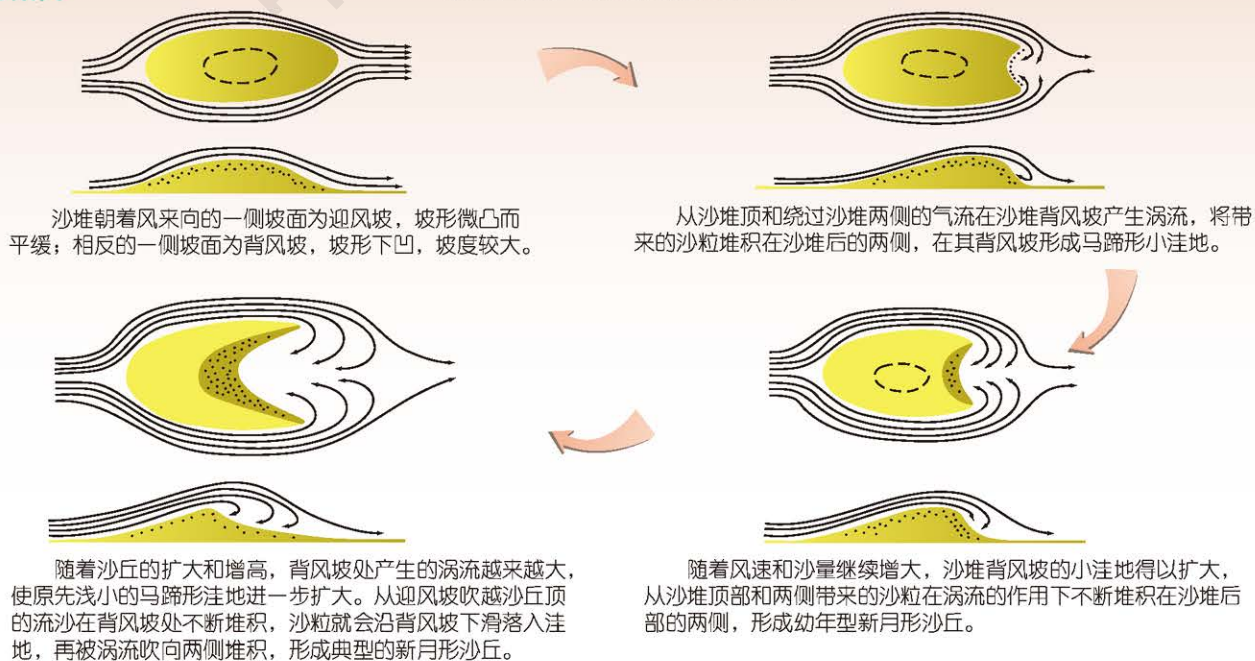
新月形沙丘形成过程示意
