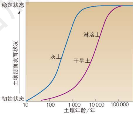
不同土壤剖面发育状况与土壤年龄关系示意
