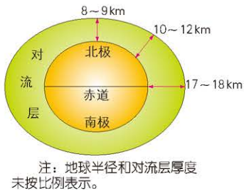
不同纬度地区对流层高度的变化
