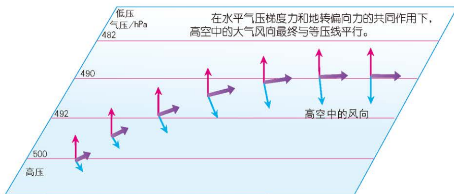
高空中风的形成示意（北半球）
