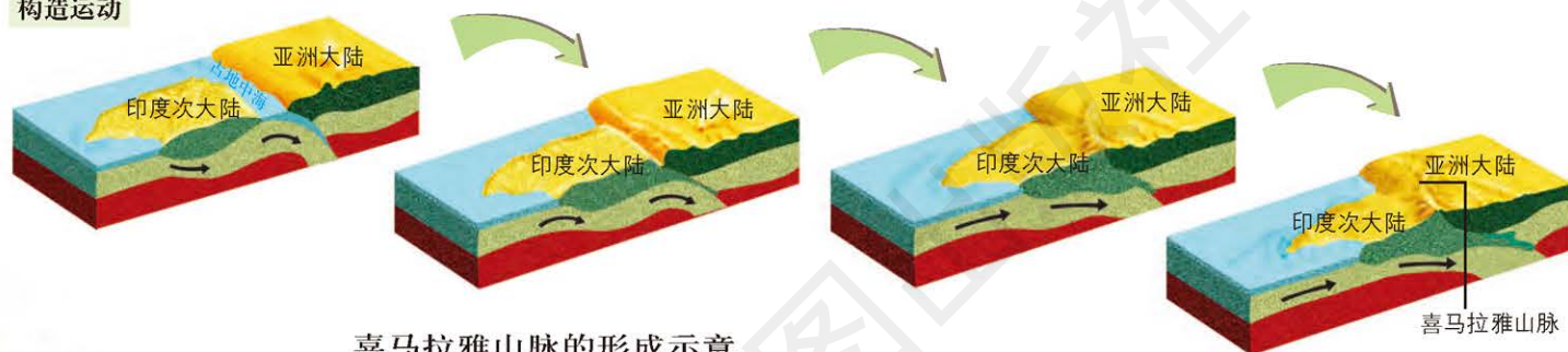
喜马拉雅山脉的形成示意
