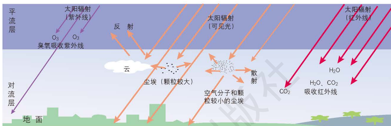
大气对太阳辐射的削弱作用
