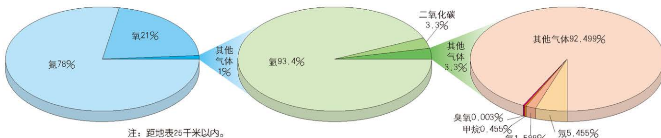
干洁空气的体积构成
