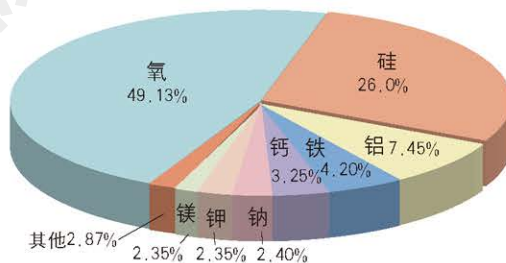
组成地壳的主要化学元素
