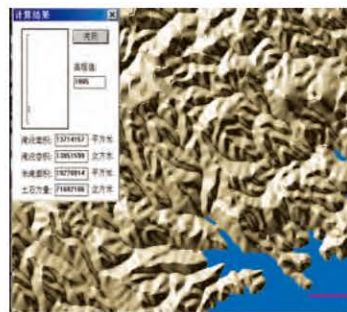
该地区可能受洪灾区域模拟图
