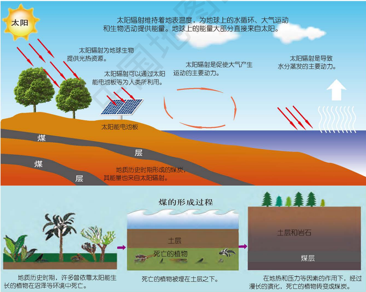
太阳辐射对地球的影响
