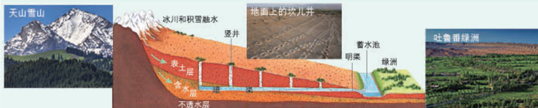
新疆坎儿井补给示意
