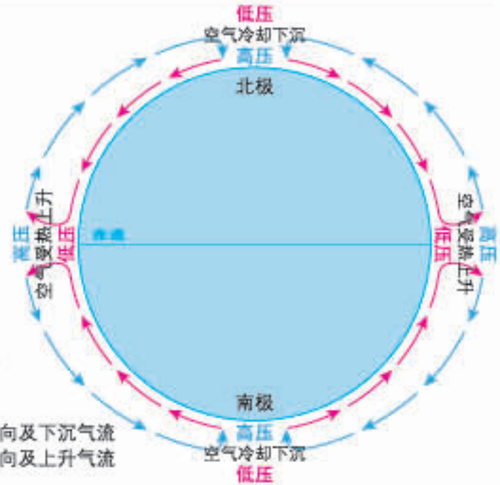
赤道与极地之间的闭合环流示意
