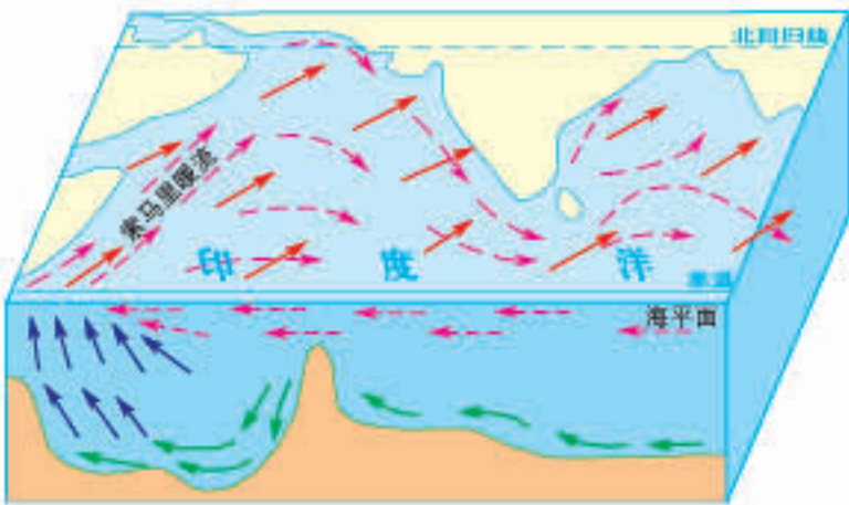
印度洋西北部海域上升流(北半球夏季)
