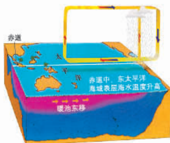
厄尔尼诺现象发生期间 大气环流示意
