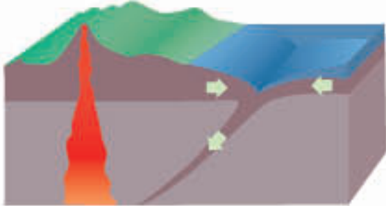
▲ 大陆板块和大洋板块碰撞，大洋板块常俯冲到大陆板块之下，形成海沟等。
