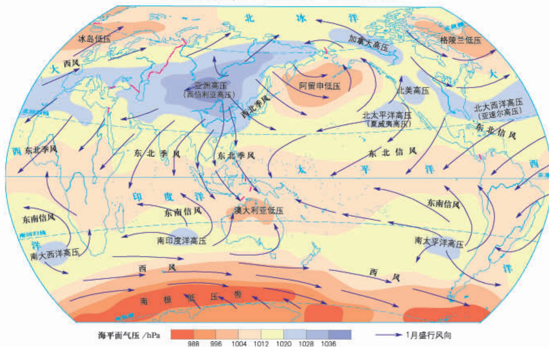
世界1月海平面气压和风 1:180 000 000
