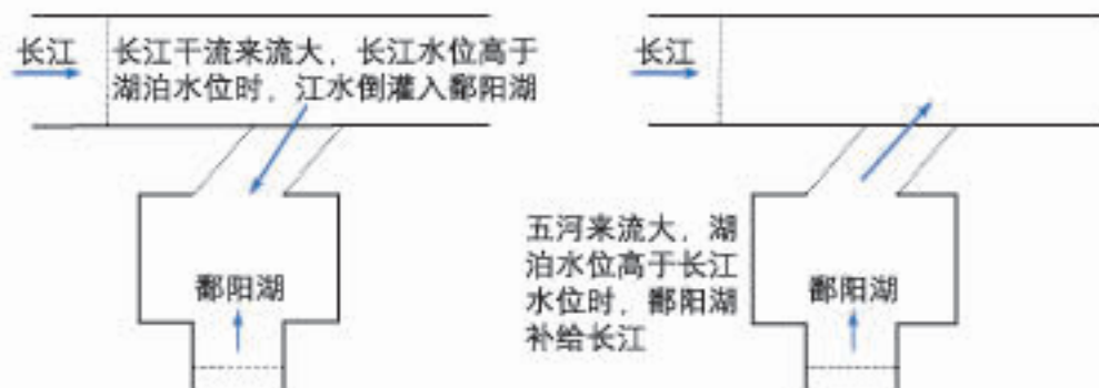
鄱阳湖与长江的相互作用示意
