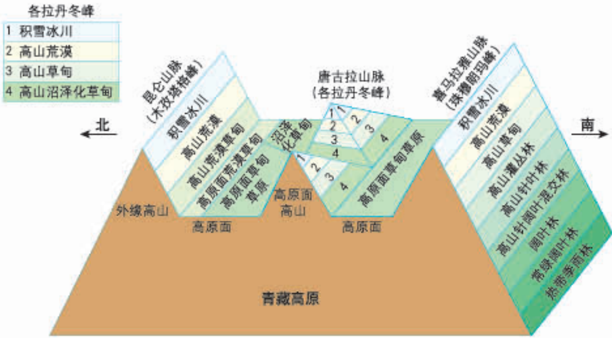
青藏高原垂直自然带
