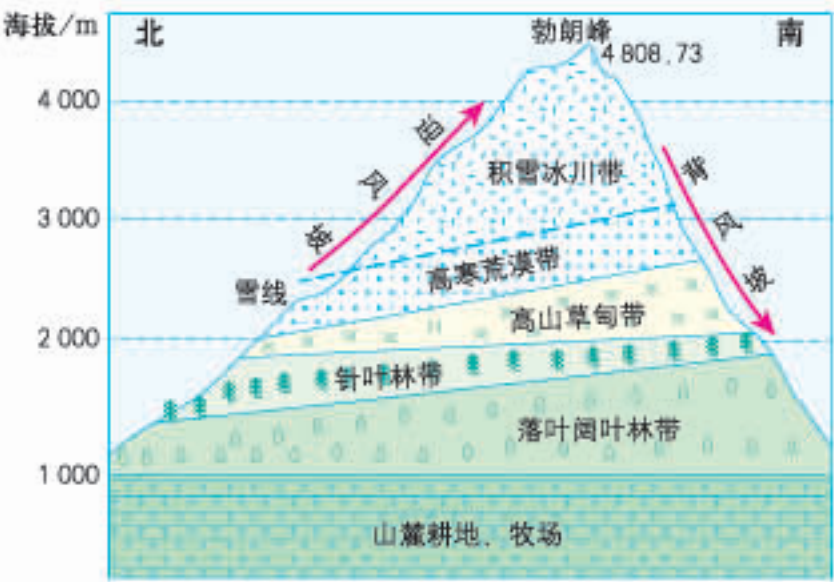
欧洲阿尔卑斯山脉的垂直自然带
