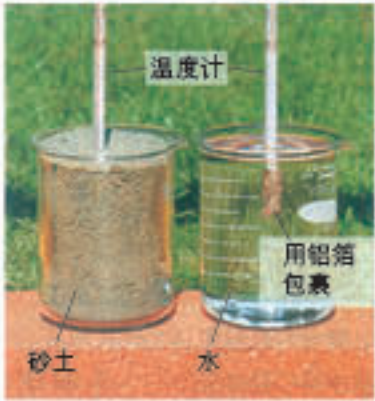
地面和水面的升温实验
