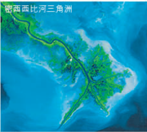
不同形态三角洲卫星影像
