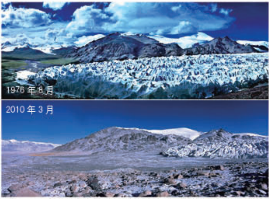
三江源区冰川退缩
