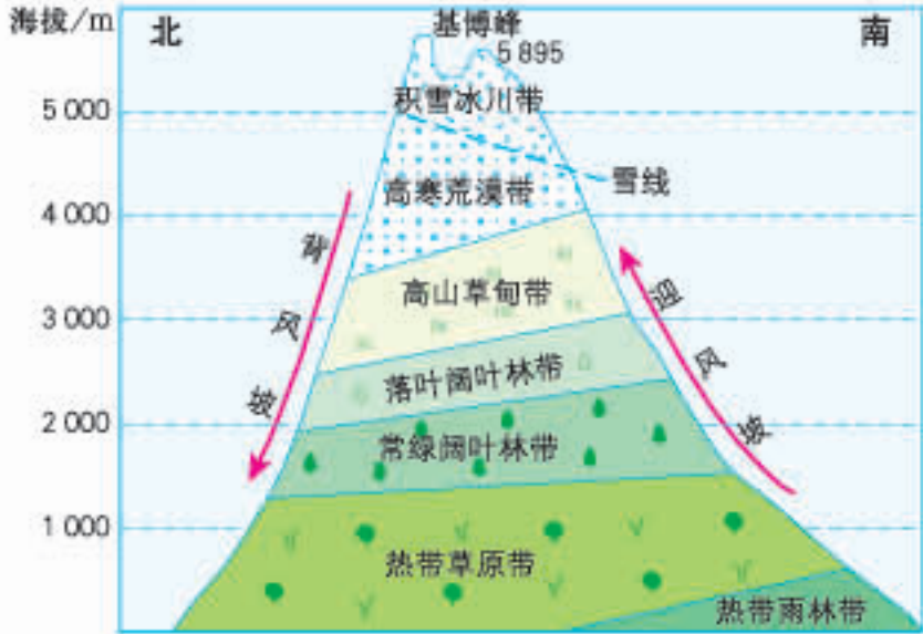
非洲乞力马扎罗山的垂直自然带
