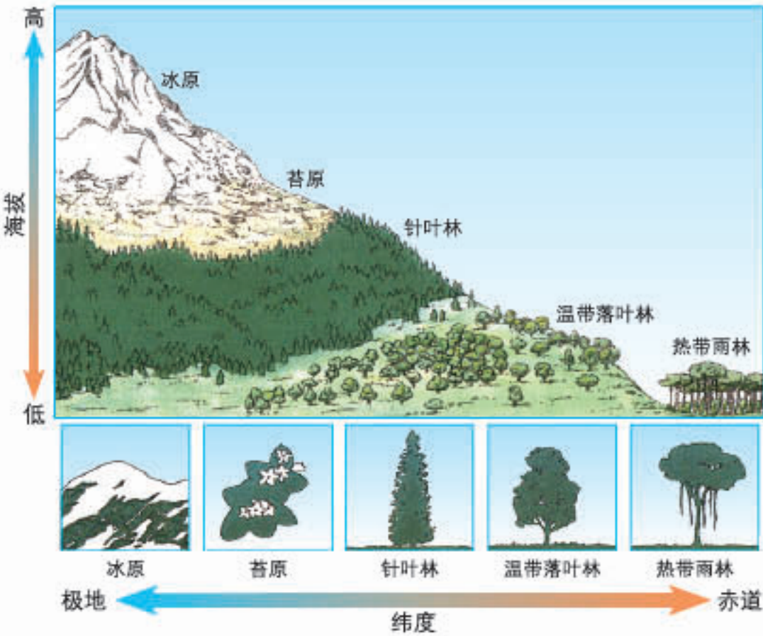
垂直分异规律与纬度分异规律的关系
