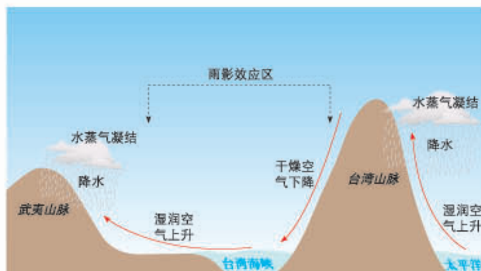
雨影效应示意
