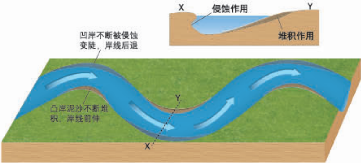
曲流河床的平面和剖面形态
