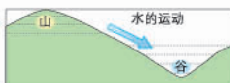
等压线与等高线
