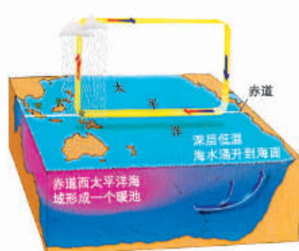
正常年份大气环流示意
