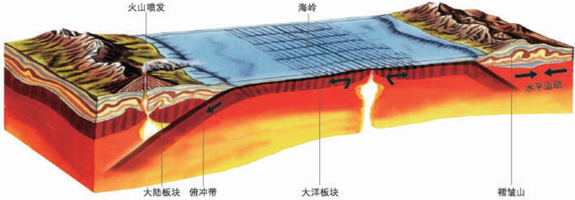
地壳运动示意
