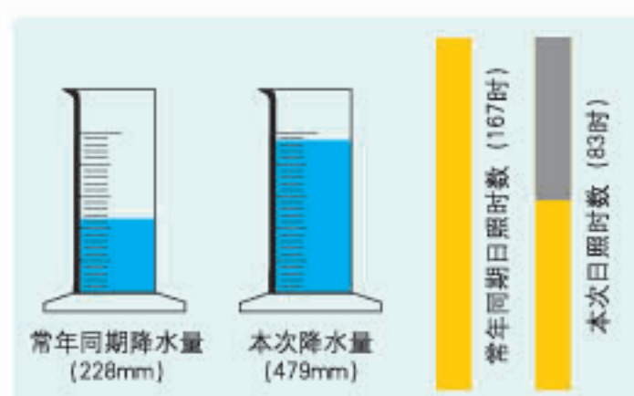
安徽省异常的降水量和日照时数 (2018年12月1日至2019年2月18日)
