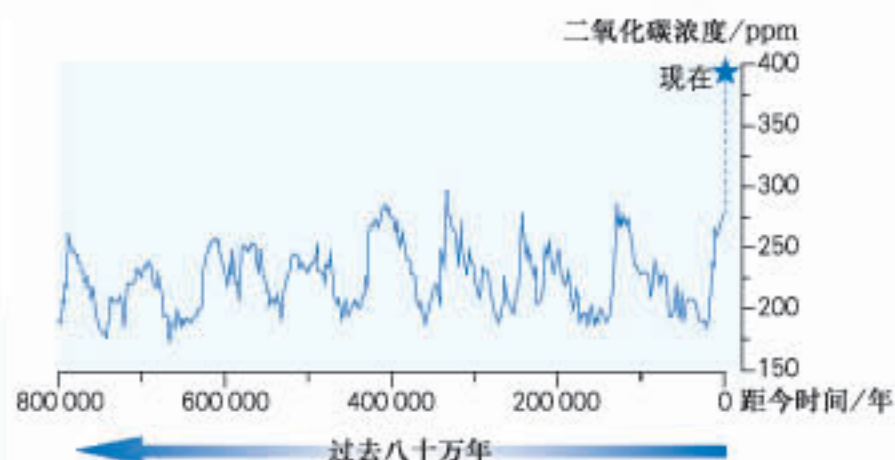
大气中二氧化碳浓度的变化
