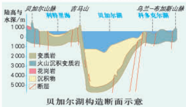
断陷湖——贝加尔湖
