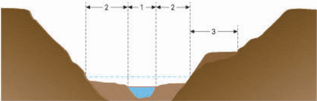
1.河床 2.河漫滩 3.阶地 — 枯水位 — 洪水位
