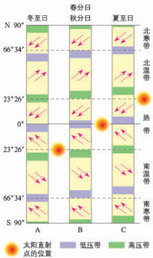
气压带和风带的季节移动示意
