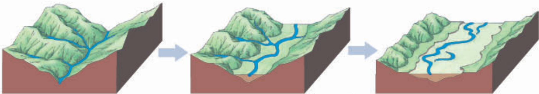
河谷的演变过程
