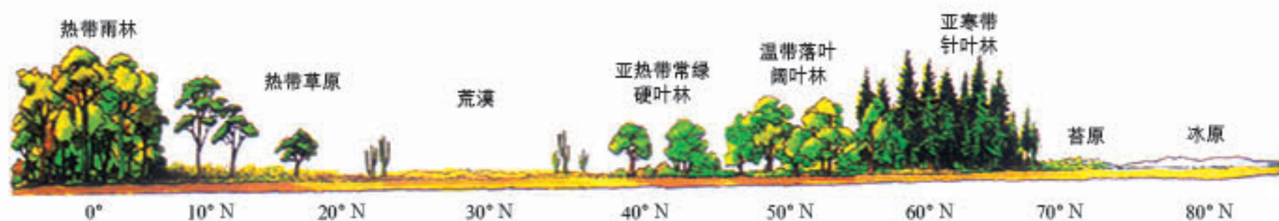
东经 20° 附近植被由赤道至北纬 80° 的变化过程
