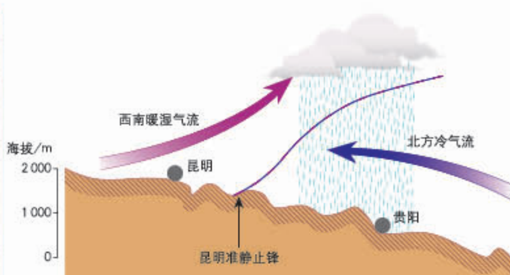
昆明准静止锋示意
