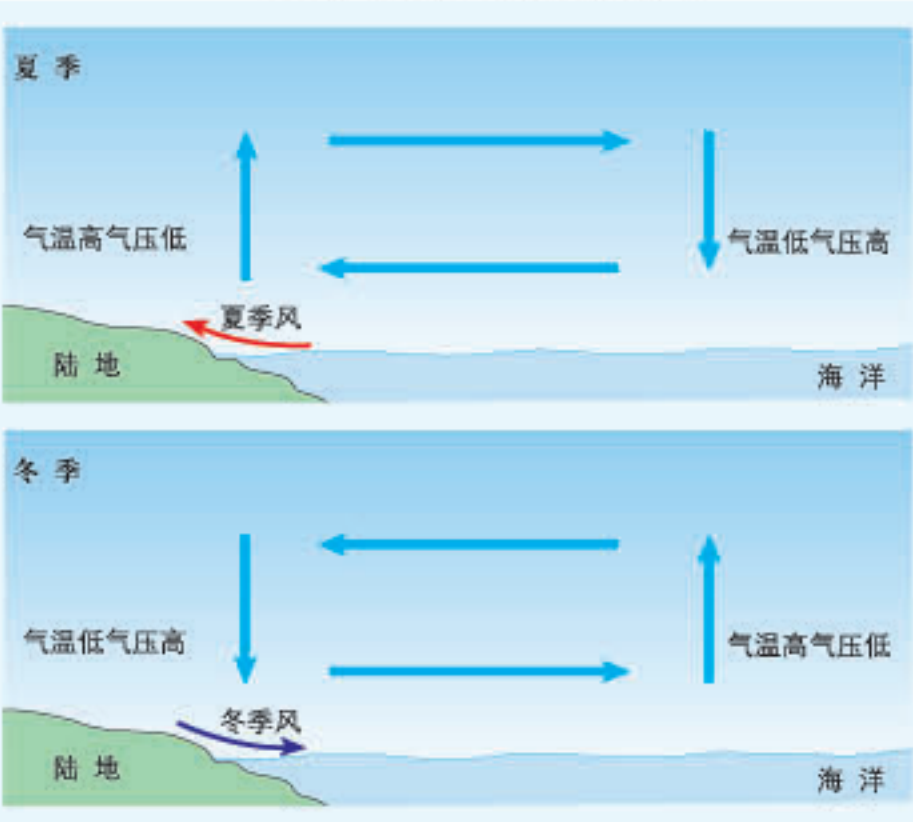
季风环流和季风成因示意
