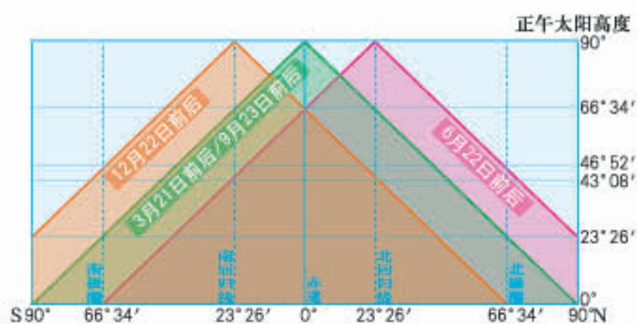
二分二至日正午太阳高度的纬度分布
