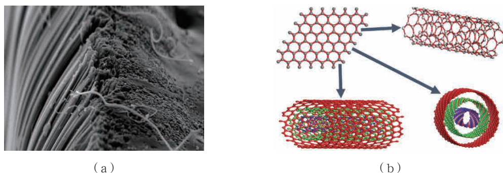
图3-3-4 一种碳纳米管的微观形貌及由石墨烯卷出碳纳米管示意图
