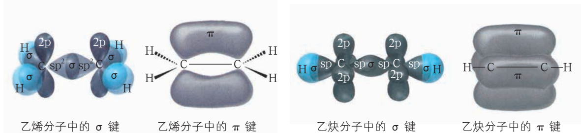
图2-2-5 乙烯分子和乙炔分子中的化学键
