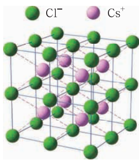
图2-3-3 氯化铯的晶体结构模型
