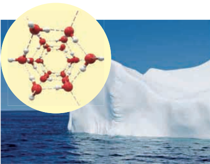
图3-2-14 冰及其微观结构
