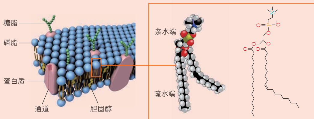
图2-2-21 细胞膜及一种磷脂的结构示意图
