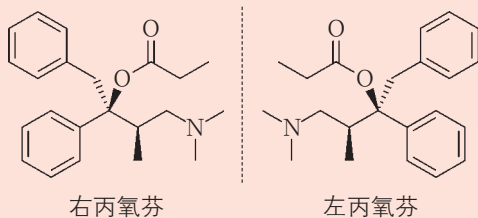
图2-2-16 右丙氧芬与左丙氧芬
