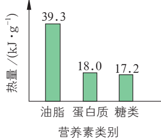
图3-3-10 1g 油脂、蛋白质、糖类完全氧化生成二氧化碳和水时放出的热量比较
