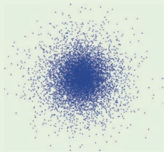
图1-1-7 氢原子的“电子云模型”
