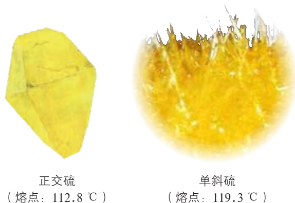
图 3-2-7 硫元素的两种同素异形体
