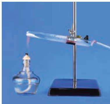
图 3-3-15 加热碳酸氢铵固体
