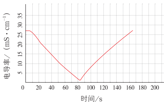
图 2-2-8 关于稀硫酸与 \text{Ba}(\text{OH})_2 溶液反应实质的研究
