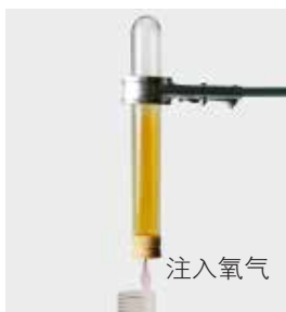
图 3-3-6 一氧化氮转化为二氧化氮
