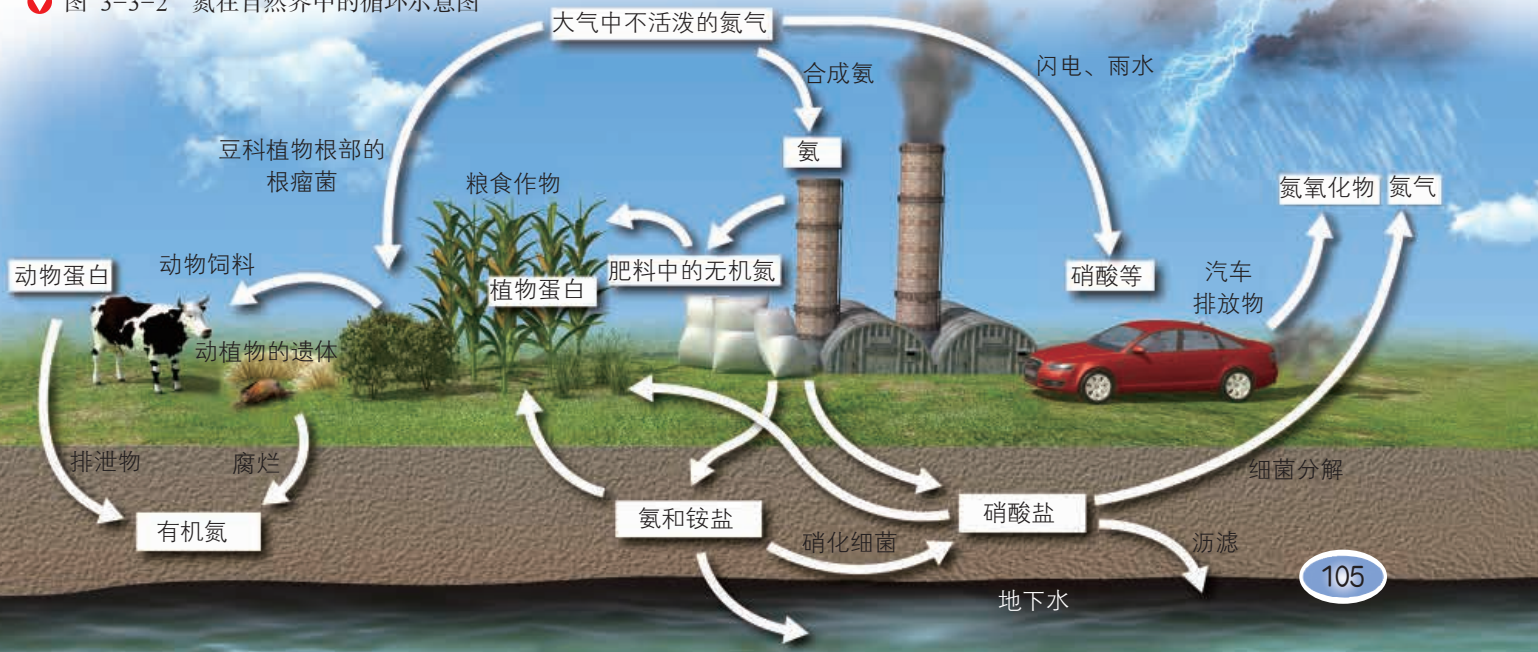
图 3-3-2 氮在自然界中的循环示意图
