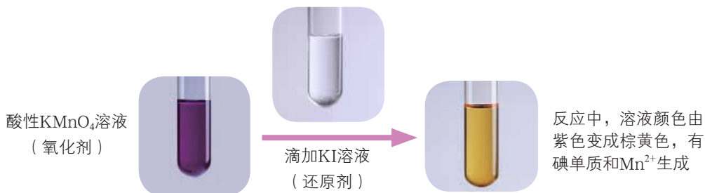
图 2-3-3 酸性 \text{KMnO}_4 溶液与 \text{KI} 溶液的反应
