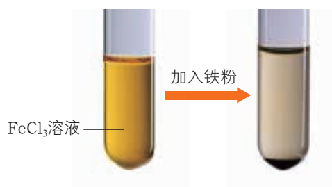
图 3-1-3 \text{FeCl}_3 溶液与铁粉的反应
