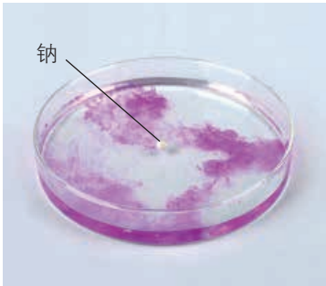
图 1-2-3 金属钠与水的反应
