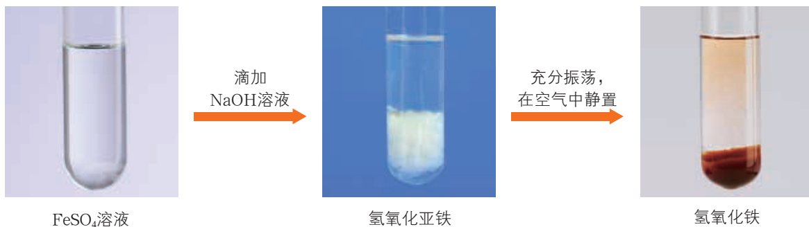
图 3-1-8 \text{FeSO}_4 溶液与 \text{NaOH} 溶液反应产生的氢氧化亚铁被空气中的氧气氧化为氢氧化铁
