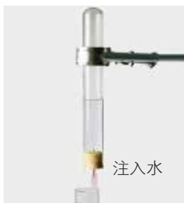
图 3-3-7 二氧化氮溶于水
