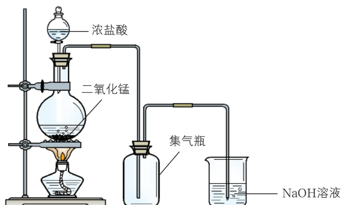
图 2-3-4 实验室制取氯气的装置示意图
