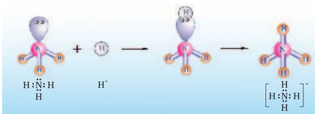
图 3-24 铵根离子形成过程示意图
