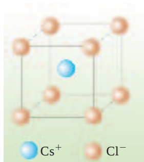
图 3-17 \text{CsCl} 晶胞结构示意图
