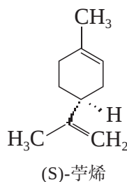
图 4-13 莰烯分子手性异构体的结构与存在
