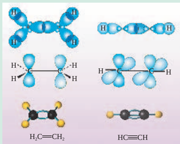
图 4-6 乙烯和乙炔的结构示意图
