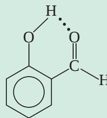
图 3-34 邻羟基苯甲醛分子内的氢键
