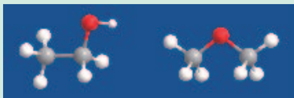
图 1-4 乙醇和二甲醚的分子结构模型
