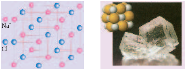
图 3-16 氯化钠晶体的结构示意图
