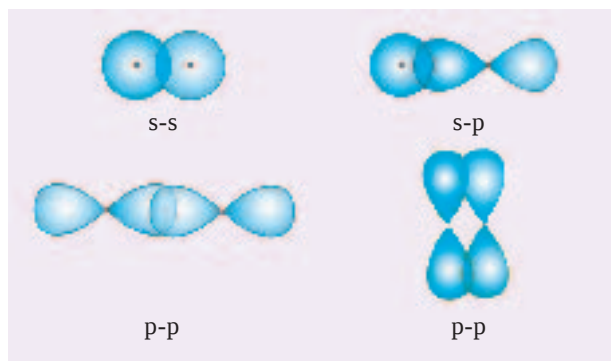
图3-20 s轨道和p轨道形成稳定共价键的几种重叠方式
