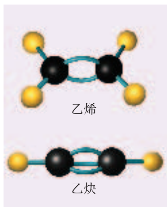
图 3-22 乙烯、乙炔分子的球棍模型
