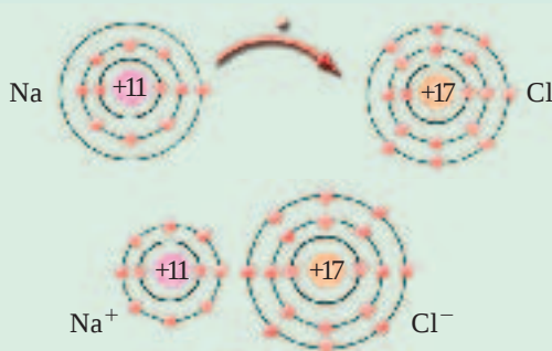
图 3-13 氯化钠中离子键的形成示意图
