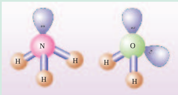
图 4-7 NH 3 分子和H 2 O分子的结构示意图
