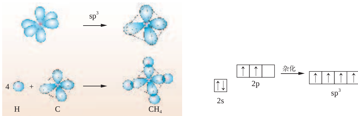
图 4-2 C原子的 \text{sp}^3 杂化轨道和 \text{CH}_4 的形成
