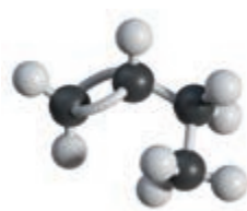
1-丁烯
