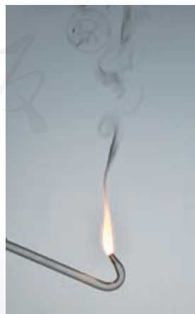
图2-7 乙炔燃烧
