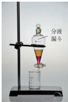
图 1-8 萃取装置
