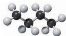
正丁烷
