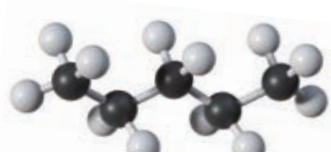
正戊烷
