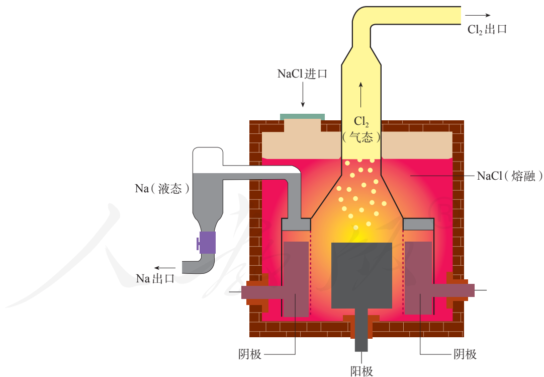
图4-16 电解熔融氯化钠装置示意图（阴极环绕在阳极外面，两极之间用隔膜隔开。在阴极区得到液态钠，在阳极区得到氯气）
