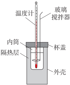
图1-3 简易量热计示意图
