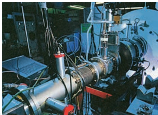
图4-6 ^{14}\text{C} 衰变测定装置（局部）
