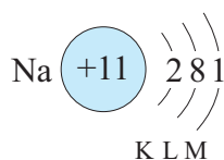
图4-2 钠原子的核外电子排布
