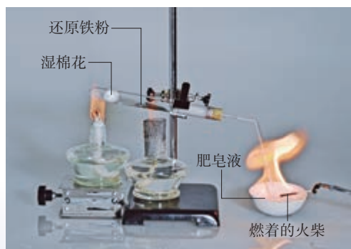
图3-5 铁粉与水蒸气反应
