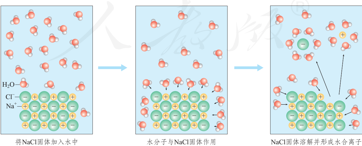
图1-11 \text{NaCl} 固体在水中的溶解和形成水合离子示意图
