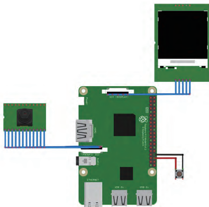
图4-14 树莓派与主要部件连接
