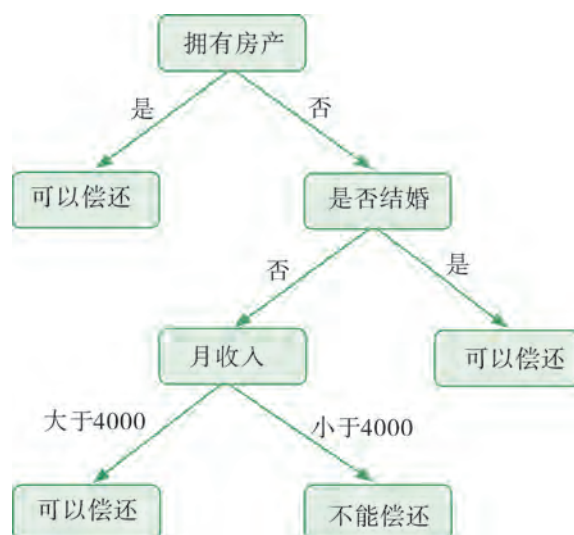
图3-9 预测用户还贷能力的简单决策树
