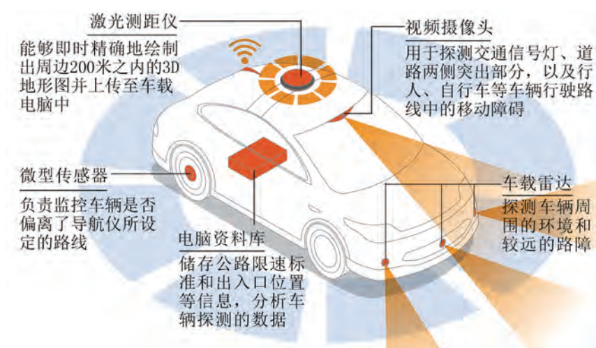
图5-4 自动驾驶汽车上的智能设备
