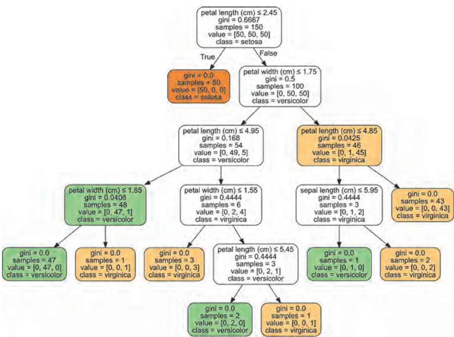
图3-11 基于鸢尾花数据集生成的决策树
