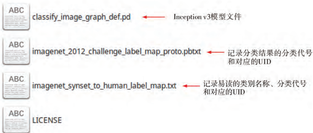
图4-11 Inception v3模型文件
