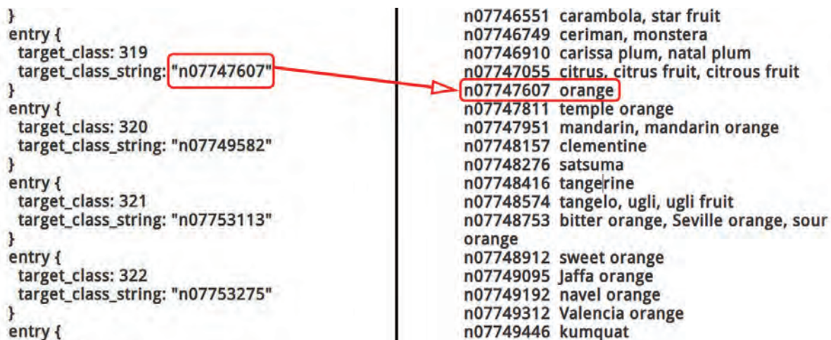
图4-12 识别结果编号与物件名称的对称关系
