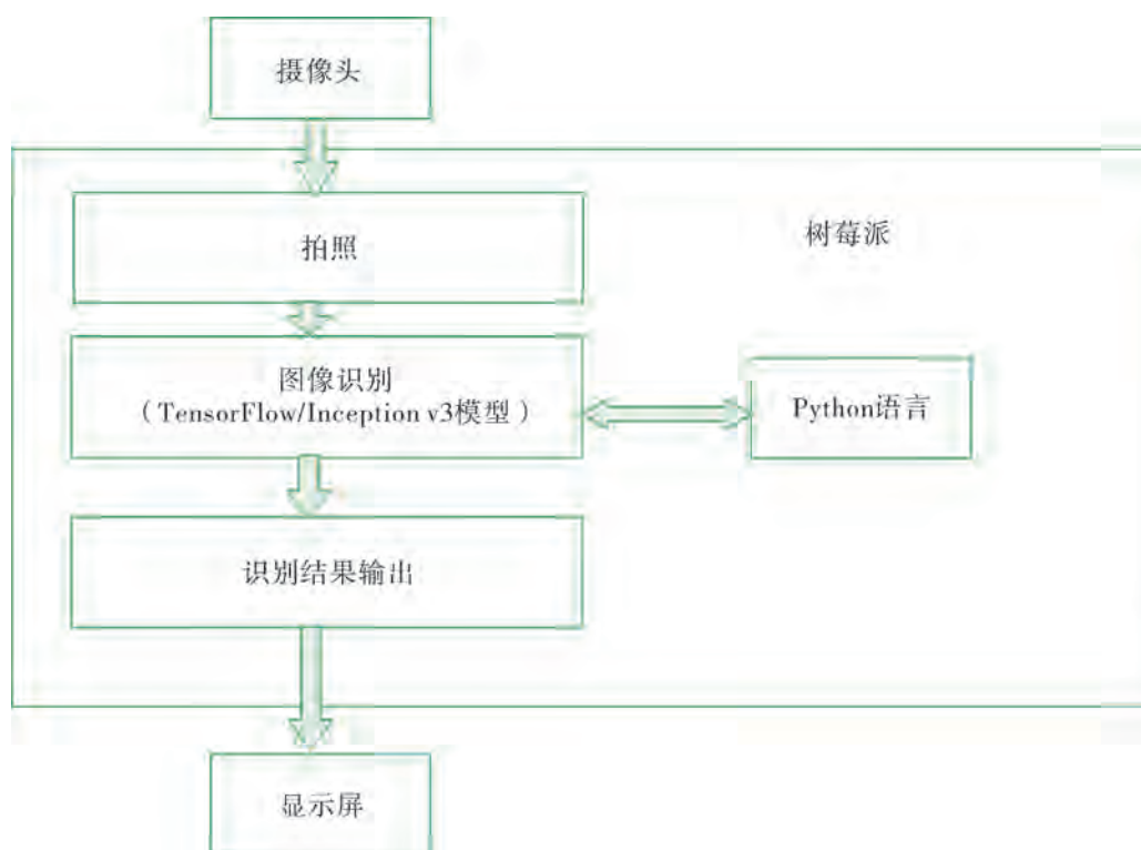
图4-8 拍照识物智能玩具系统软件模块设计示意图
