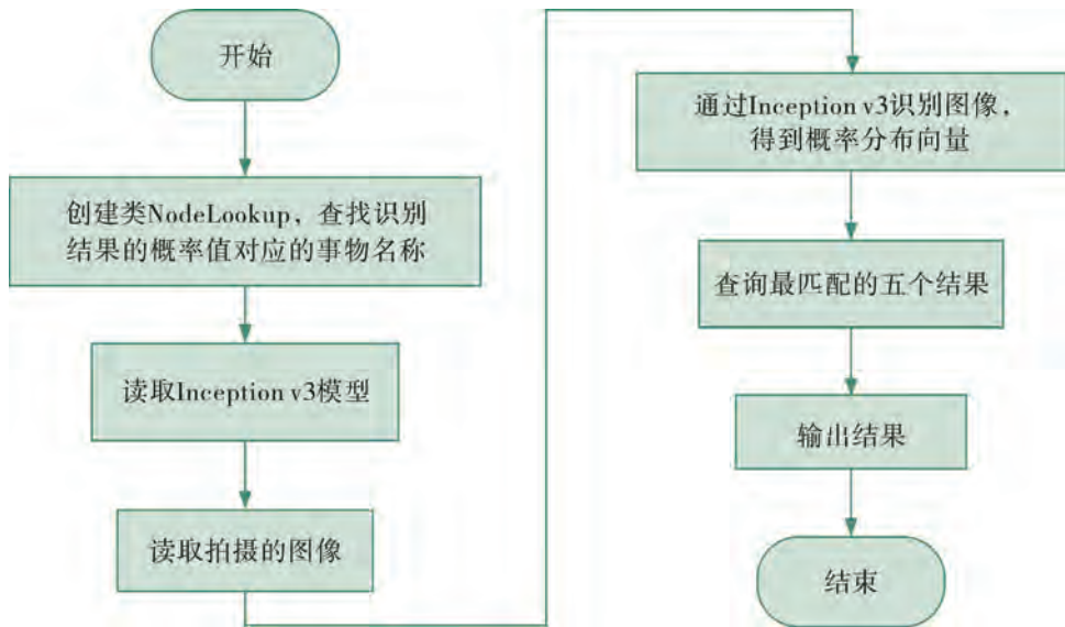
图4-10 图像识别应用模块程序实现流程图
