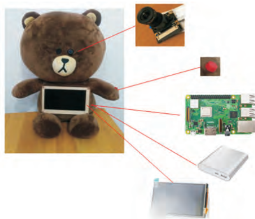
图4-13 拍照识物智能系统玩具集成
