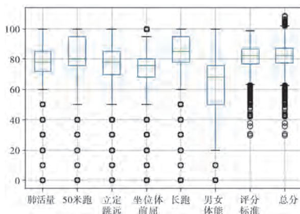
图4-27 测试项目得分箱形图
