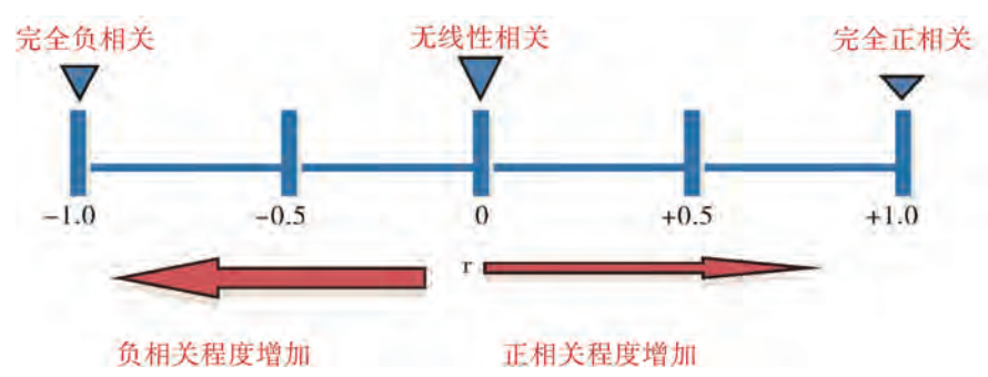
图4-19 皮尔逊相关系数指标
