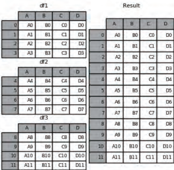
图4-10 纵向合并数据
