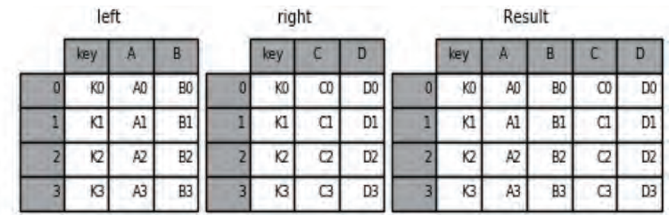
图4-14 执行结果示意图
