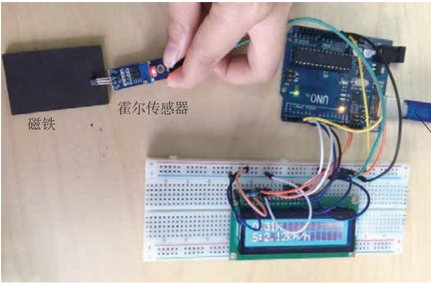
图 2-42 测试自行车里程仪
