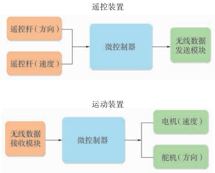
图 3-21 无人船模型系统结构图
