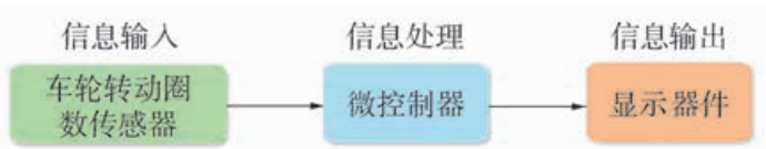
图 2-30 自行车里程仪初步设计图
