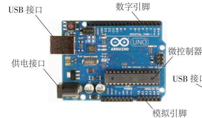
图 1-10 UNO 板
