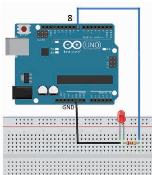
图 1-19 一个 LED 的控制电路图
