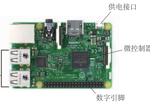
图 1-11 树莓派
