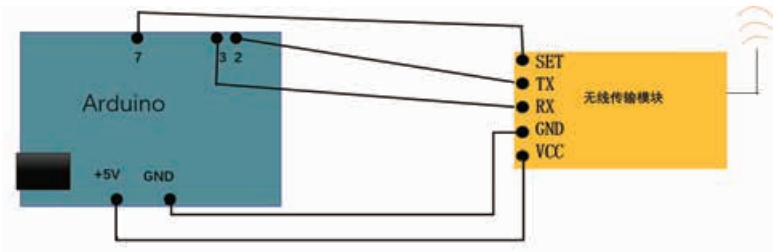
图 3-8 发射端连线图
