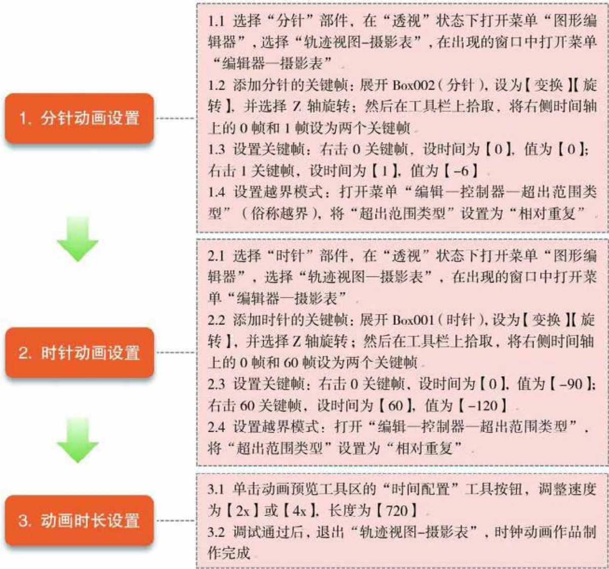
图 3-23 时钟走动动画的动画制作流程
