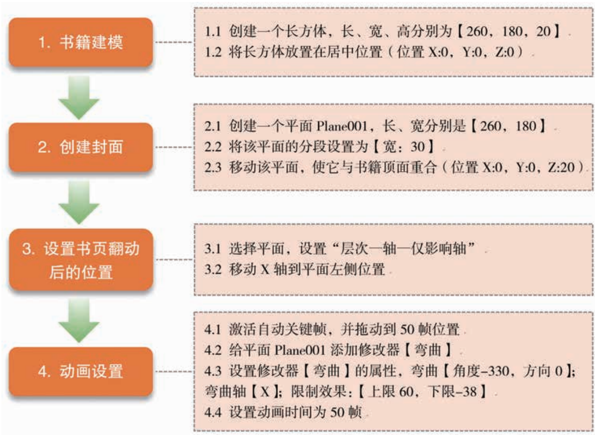
图 3-25 书页翻动动画制作流程
