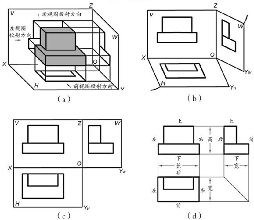
图 2-15 三视图投影规律
