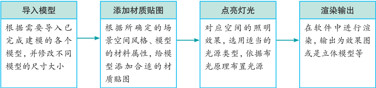
图 2-44 优化模型的一般流程
