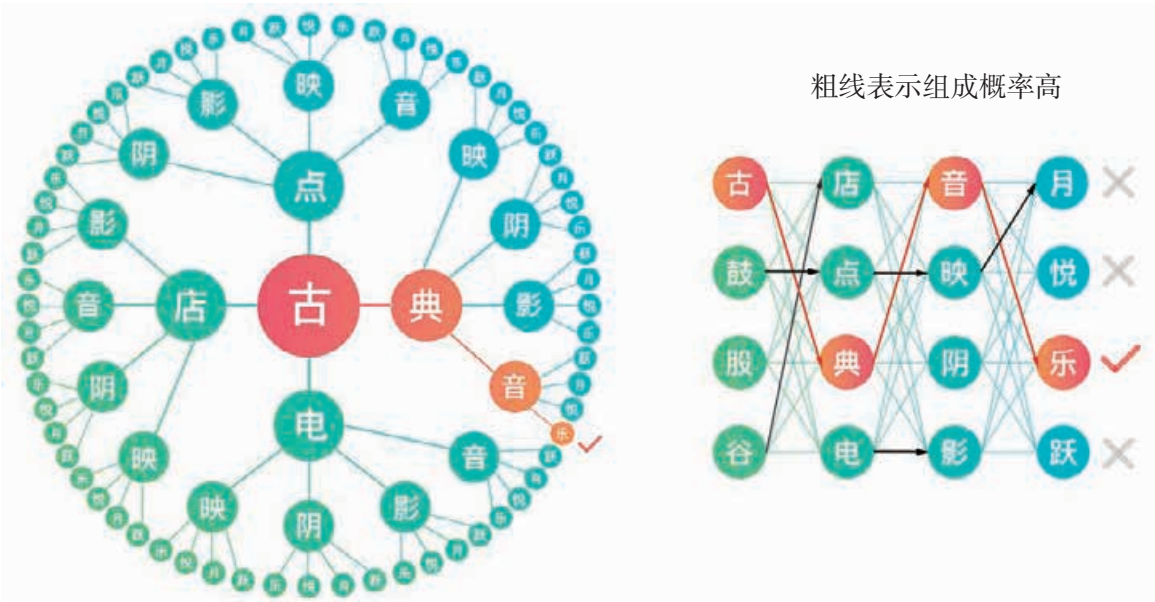
图 2-38 穷举（左）和 Viterbi 算法（右）在四个隐含节点下的计算量
