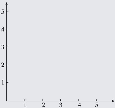
图 2-94 二维坐标系
