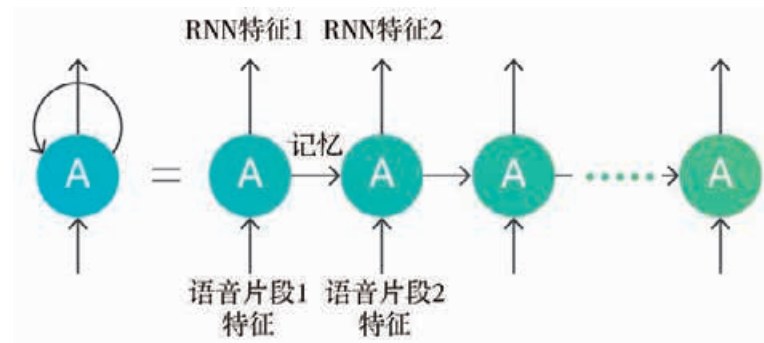
图 2-41 RNN 结构
