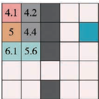
图 2-59 使用 A* 算法搜索最短路径之 3
