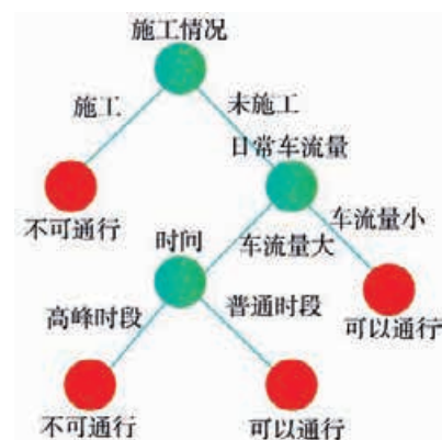
图 2-49 决策树示例
