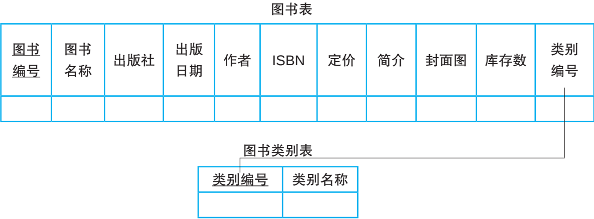
图 2-16 表间联系示意
