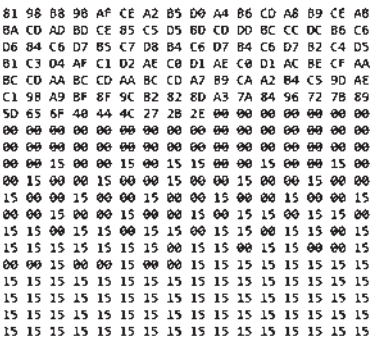
图 2-10 某应聘者照片的部分图像数据
