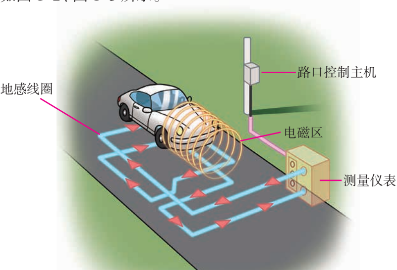
图 1-2 利用地感线圈采集数据
