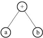
图 4-5 a+b 的表达式二叉树
