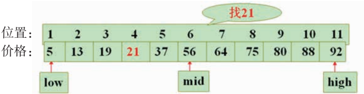
图 5-8 有序的商品价格序列
