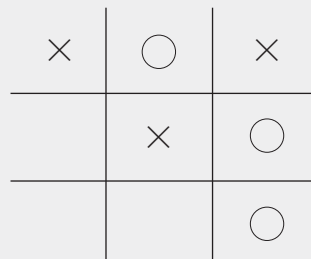
图 2-3 井字棋, 格局
