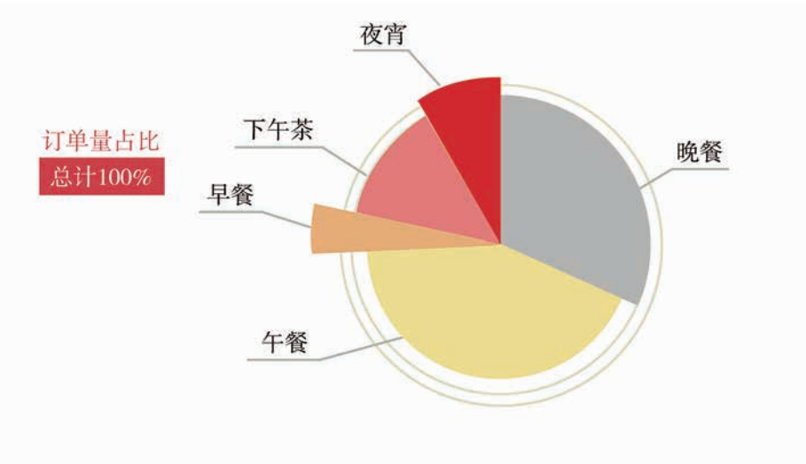
图 1-13 订单量占比
