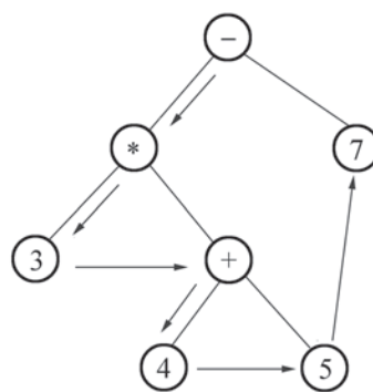
图 4-4 先序遍历
