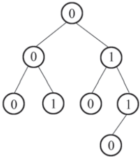
图 4-13 二叉树
