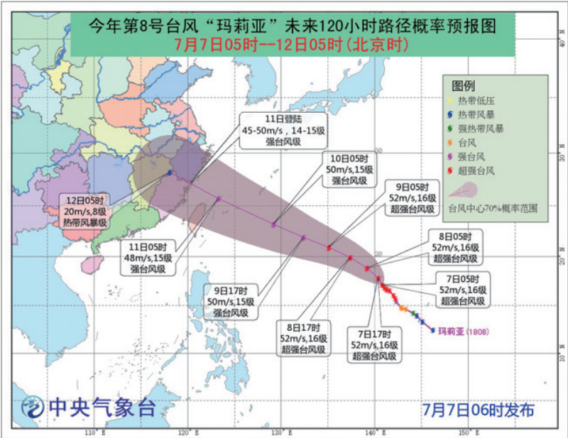
图 1-4 台风路径概率预报图
