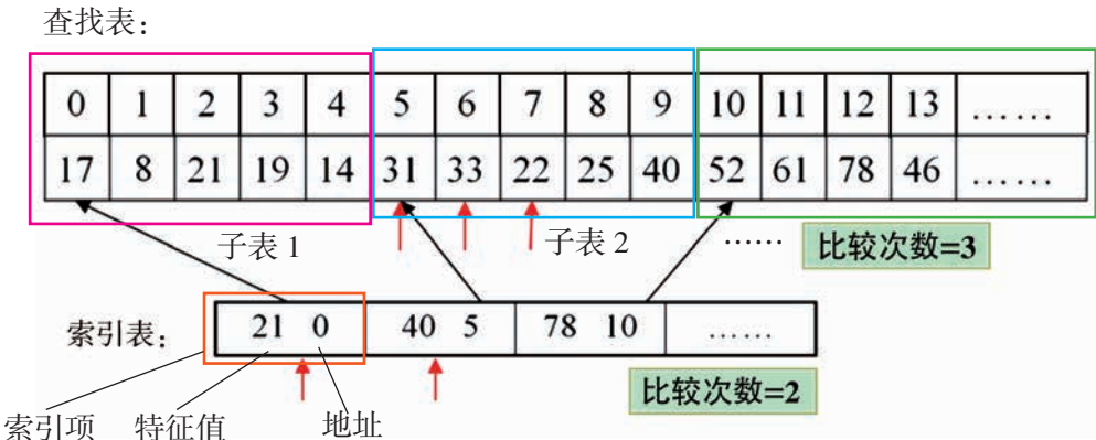
图 5-13 索引表
