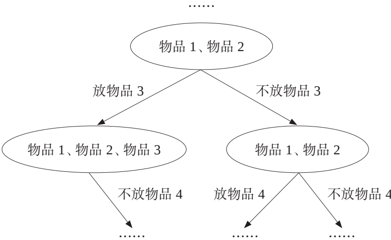
图 4-12 示例
