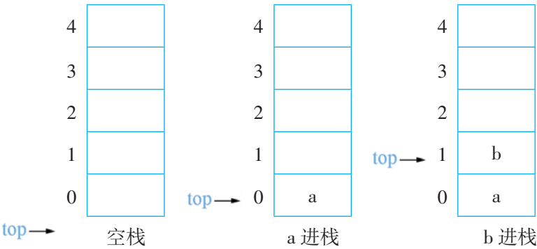
图 3-9 进栈示意
