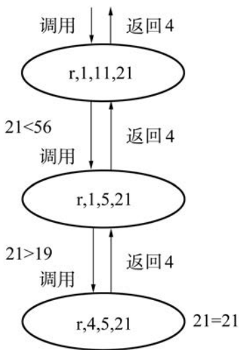
图 5-12 递归调用与返回
