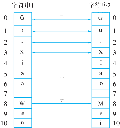
图 3-18 比较过程
