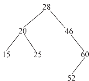
图 5-16 二叉树
