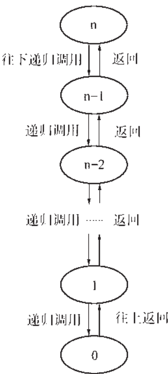
图 5-15 递归状态图
