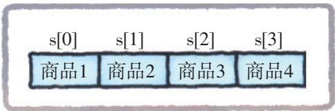
图 2-9 数组
