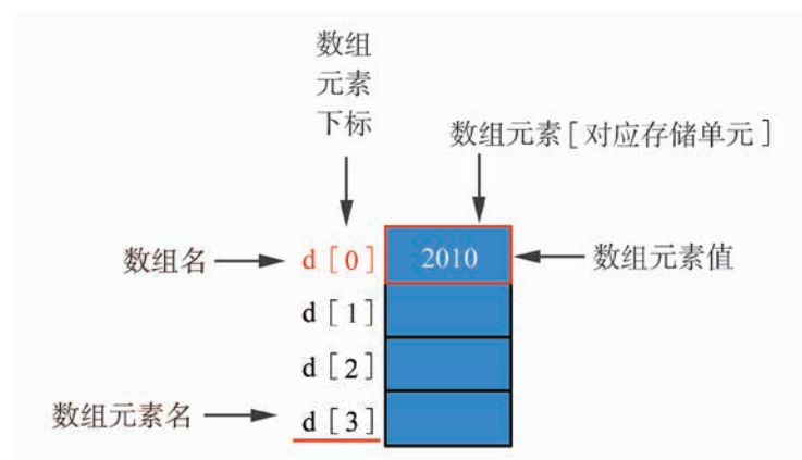
图 2-16 数组 d
