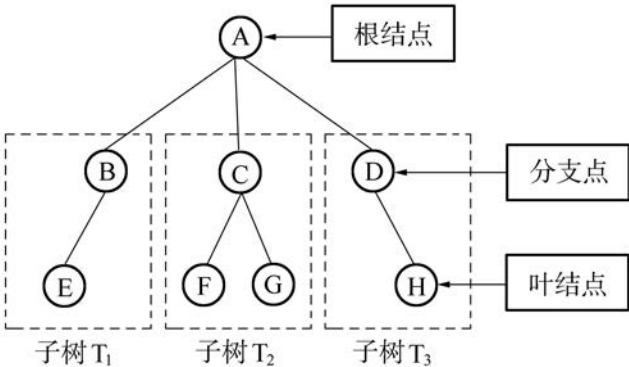
图 4-9 树示例
