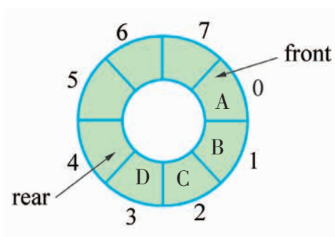
图 3-5 循环队列
