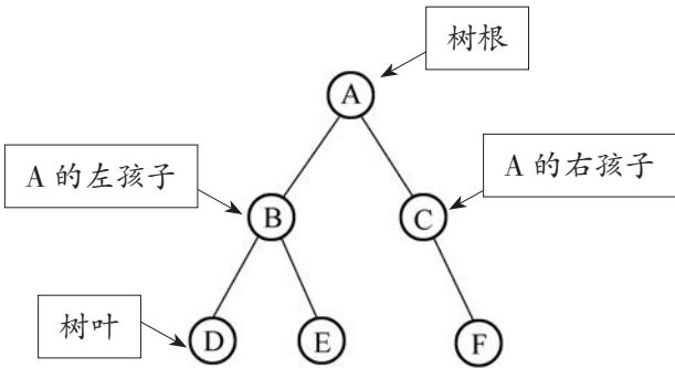
图 4-10 二叉树示例
