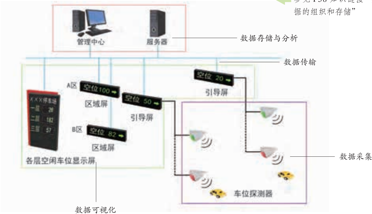
图 2-30 停车引导中的数据处理
