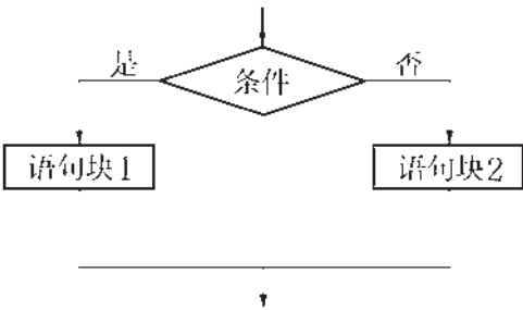
图 3-32 双分支结构
