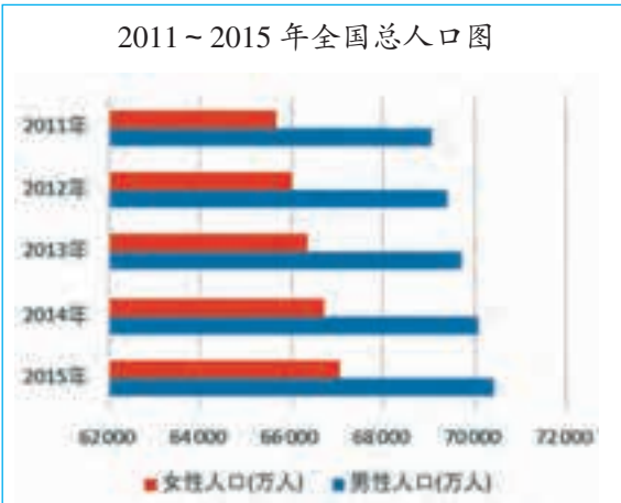
图 2-18 条形图示例
