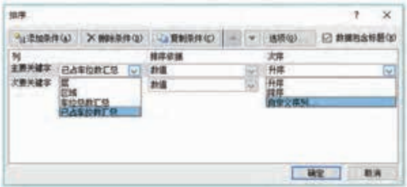
图 2-37 排序工具
