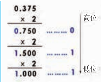
图 1-24 小数部分的转换
