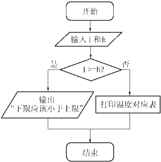
图 3-17 打印温度对应表的流程图
