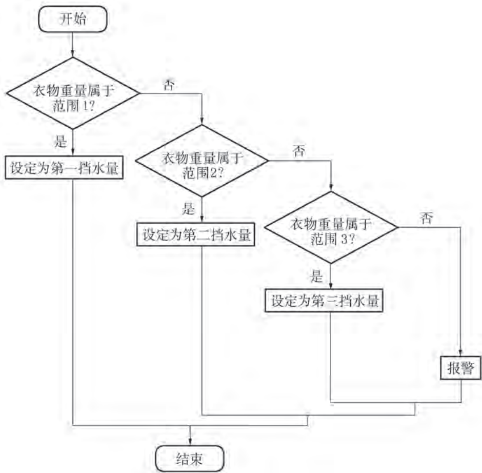
图 3-8 自动设定水位的流程图
