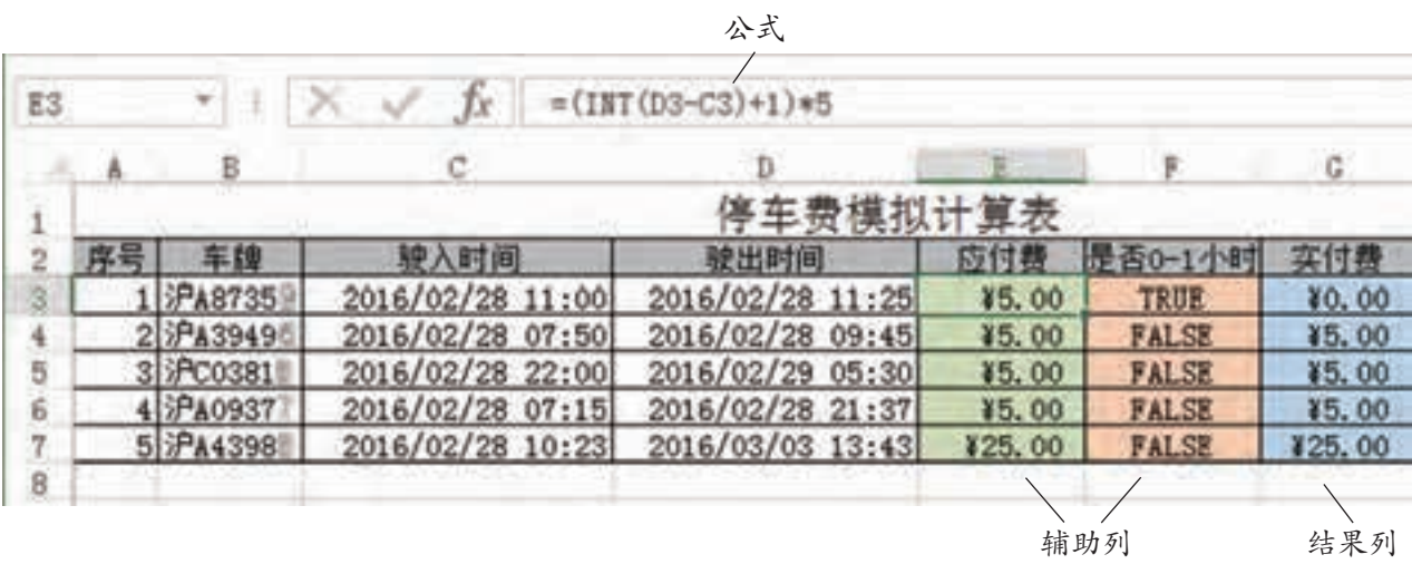
图 2-33 停车费模拟计算表
