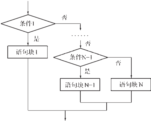
图 3-33 多分支结构
