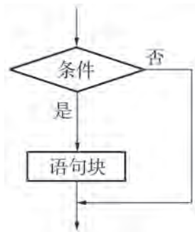
图 3-31 单分支结构
