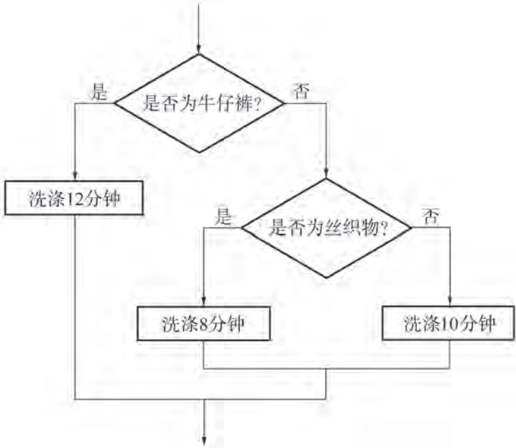
图 3-5 设定洗涤时长的流程图
