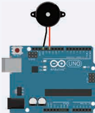
图 2.26 音乐播放器实物连接图
