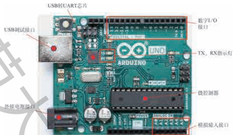
图 1.17 A rdu ino Uno 开发板的组成
