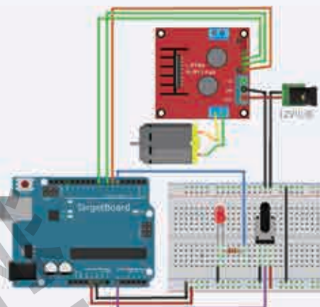
图 2.36 调速小风扇实物连接图
