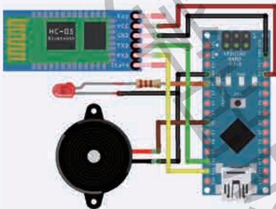
图 3.18 蓝牙模块与 Arduino Nano 连接图
