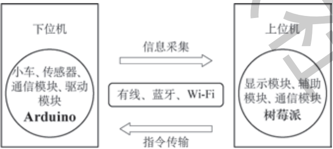
图 4.2 小车控制实现示意图
