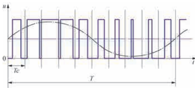
图 2.28 PWM 示意图
