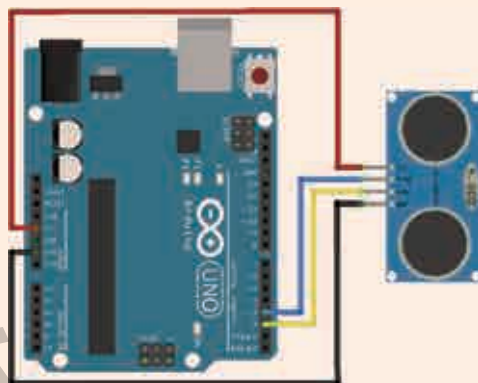
图 2.22 超声波测距各模块连接图
