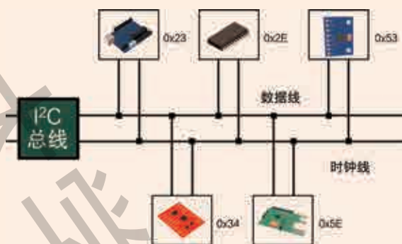
图 3.9 I 2 C 模块在 I 2 C 总线上的连接示意图
