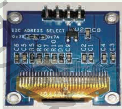
图 3.10 I 2 C 接口的 OLED 模块
