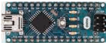
图 1.18 A rdu ino Nano 开发板
