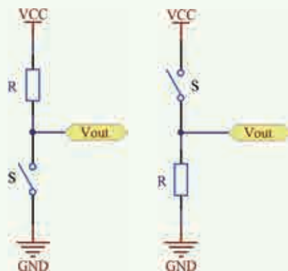
图 2.7 上拉电阻连线
