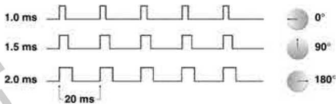
图 2.34 舵机的旋转角度控制
