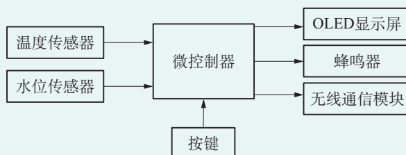
图 1.43 智能水杯电子控制系统设计框图
