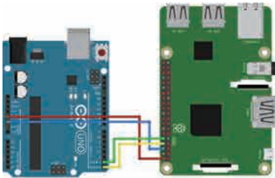
图 4.26 树莓派与 Arduino通过 GPIO 接口连接的实物搭建图
