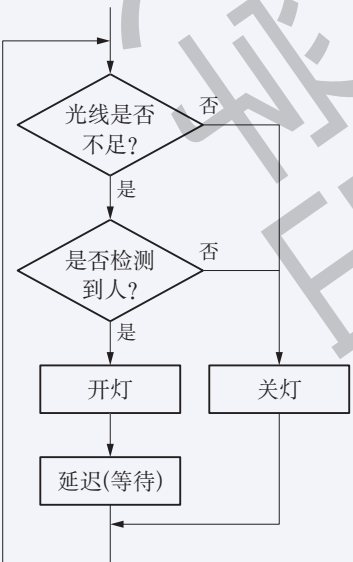
图 2.18 感应节能夜灯流程示意图
