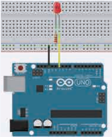
图 2.30 呼吸灯实物连接图
