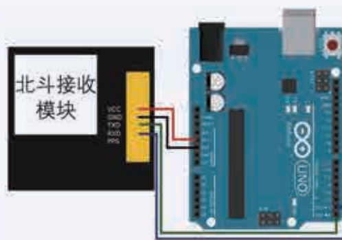
图 3.5 Arduino Uno与北斗接收模块连接图
