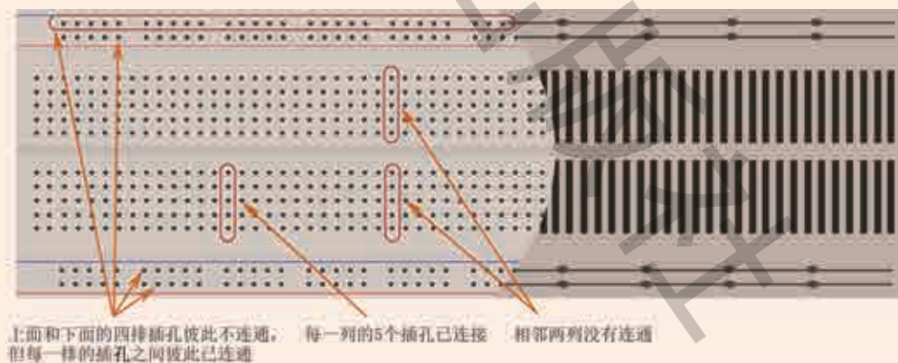
图 2.11 面包板正反面对比图
