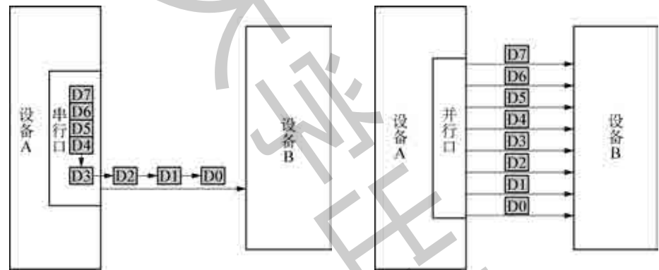
图 3.2 串行通信示意图
