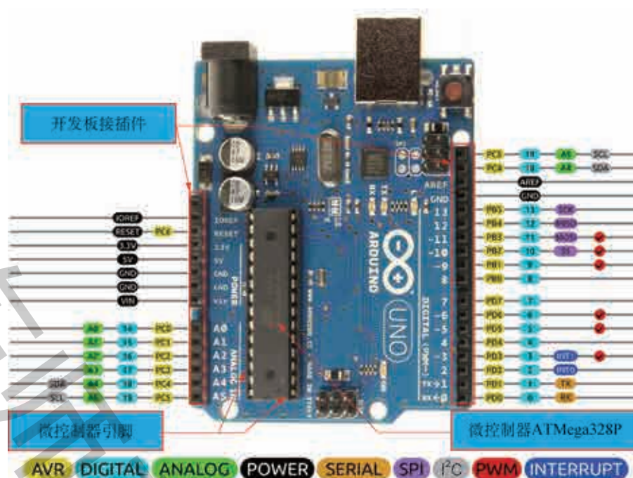
图 2.3 Arduino Uno 引脚和引脚复用功能示意图
