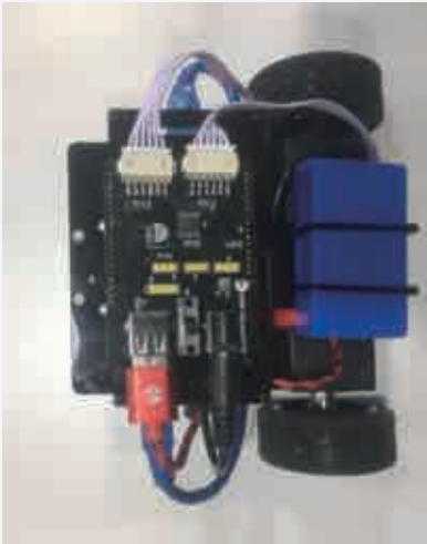
图 4.5 运动小车的完整组装
