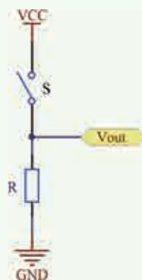
图 2.8 下拉电阻连线
