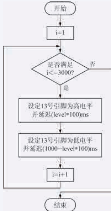
(b) 根据 level 值设定占空比并输出高低电平
