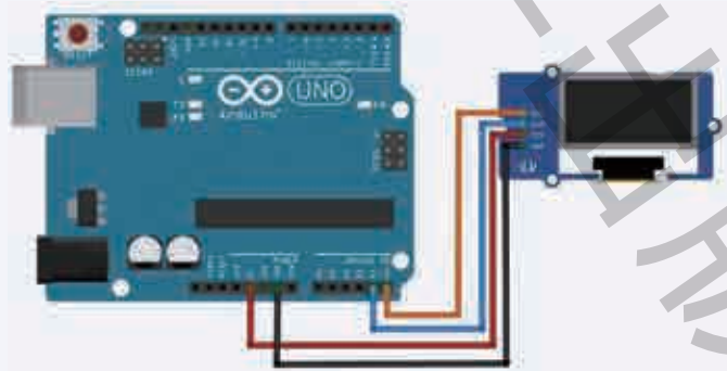
图 3.11 Arduino Uno 与 OLED 模块连接图
