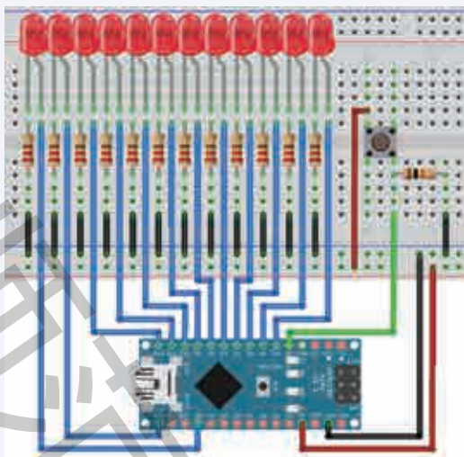
图 2.46 安全警示灯实物连接图
