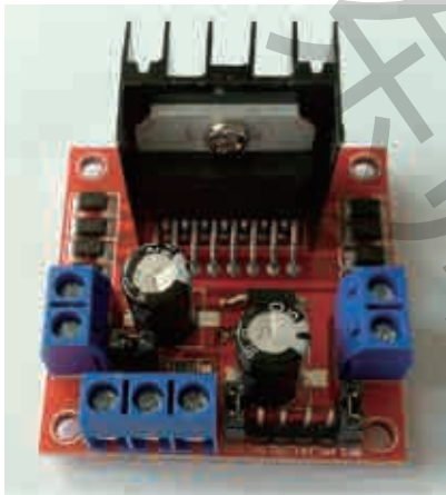
图 2.31 L298N 电机驱动模块
