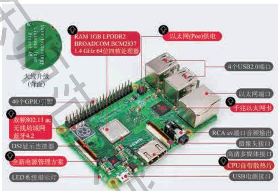
图 1.24 树莓派 3B+ 开发板
