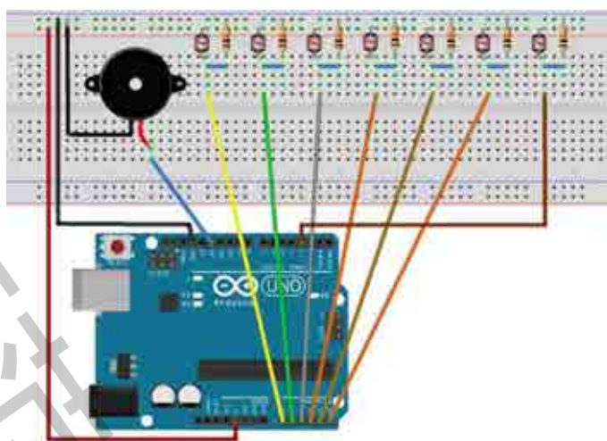
图 2.27 光敏电子琴
