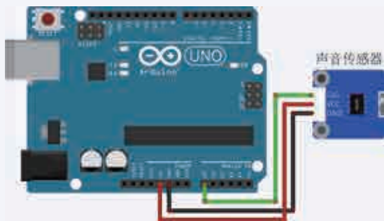
图 2.15 机器耳朵实物连接图
