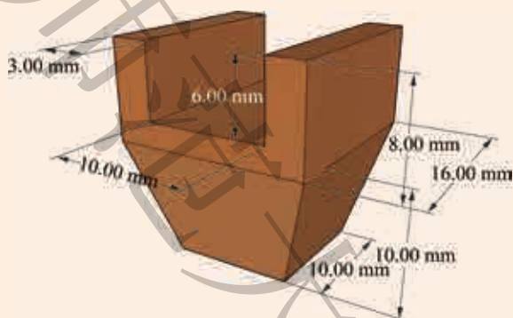
图 2.29 “斗”的参考尺寸
