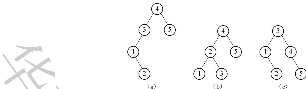
图 5.12 二叉搜索树的平衡操作
