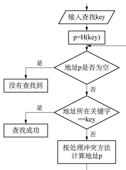
图 4.20 查找流程图
