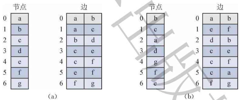
图 4.13 图的两计算机表示方法
