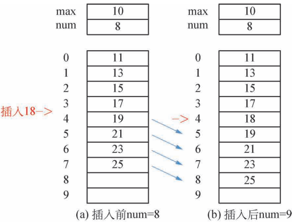
图 3.5 顺序表插入前后的情况
