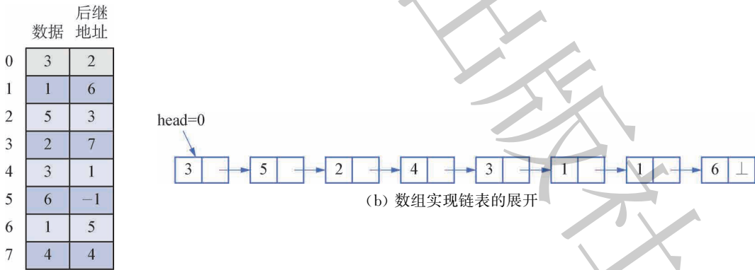
图 3.8 用二维数组实现链表 (a) 用数组实现链表
