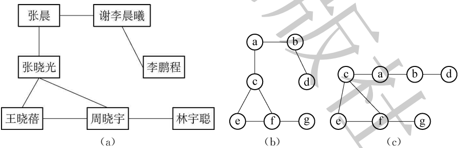
图 4.12 图的示例
