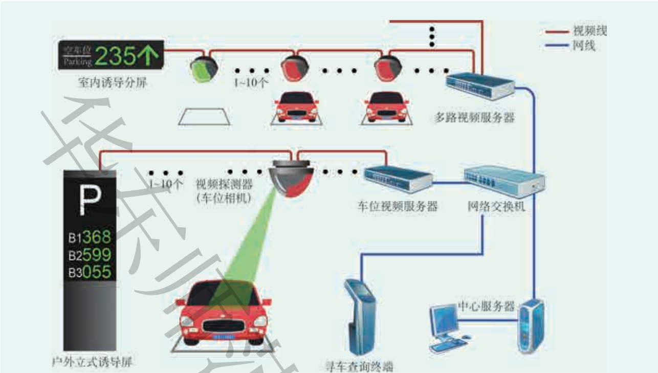
图 2.1 智能停车场内部设备示意图
