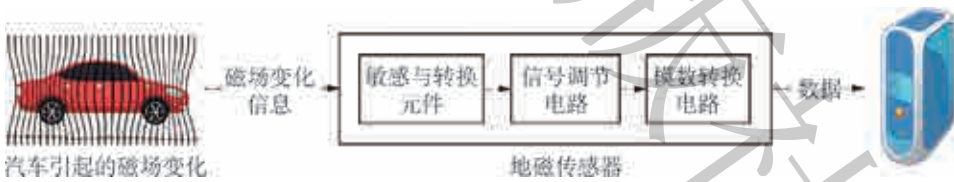
图 2.17 地磁传感器的信息转换过程
