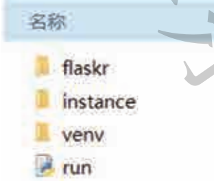
图 3.23 myproject 文件夹
