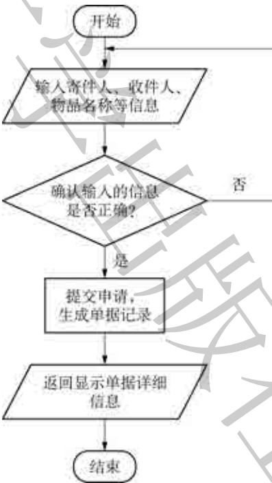
图 3.21 下单流程图
