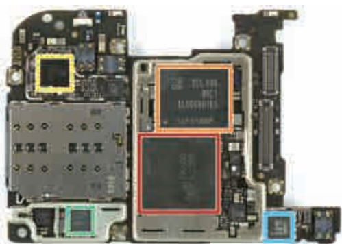
图 2.8 某智能手机主板
