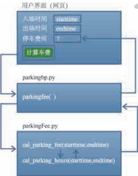
图 2.40 程序调用过程示意图
