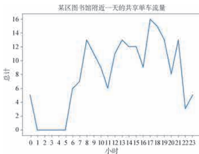
图 3.23 绘制折线图
