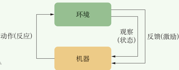
图 4.23 强化学习
