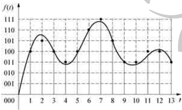
图 1.19 量化
